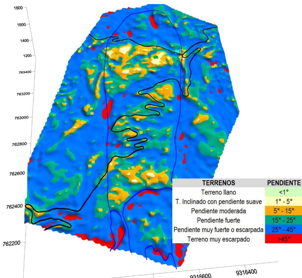
Figura 4. Modelo 3D de las pendientes del terreno afectado por reptación (en línea azul) en el caserío Musungate utilizando el MDE obtenido con el levantamiento fotogramétrico.
