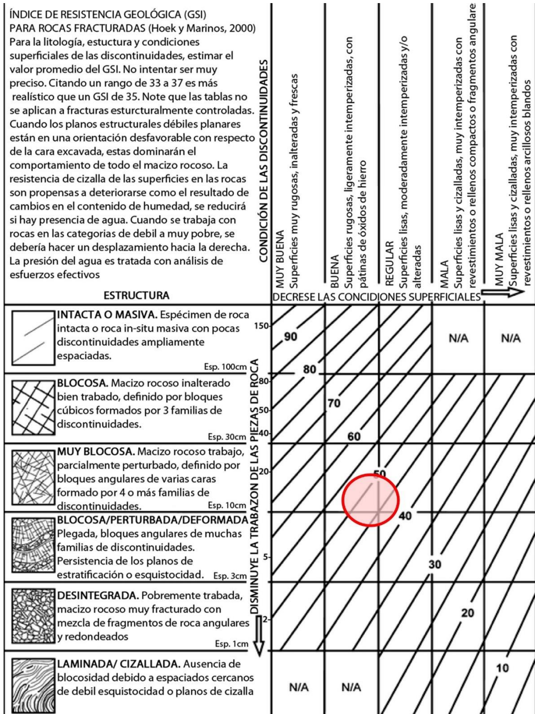
Gráfico 2. Estructura y calidad de las discontinuidades de los macizos rocosos de la Formación Oyotún (Jm-o), GSI promedio de 48. Fuente: Tabla del Índice Geológico de Resistencia GSI (Hoek, 2007).
