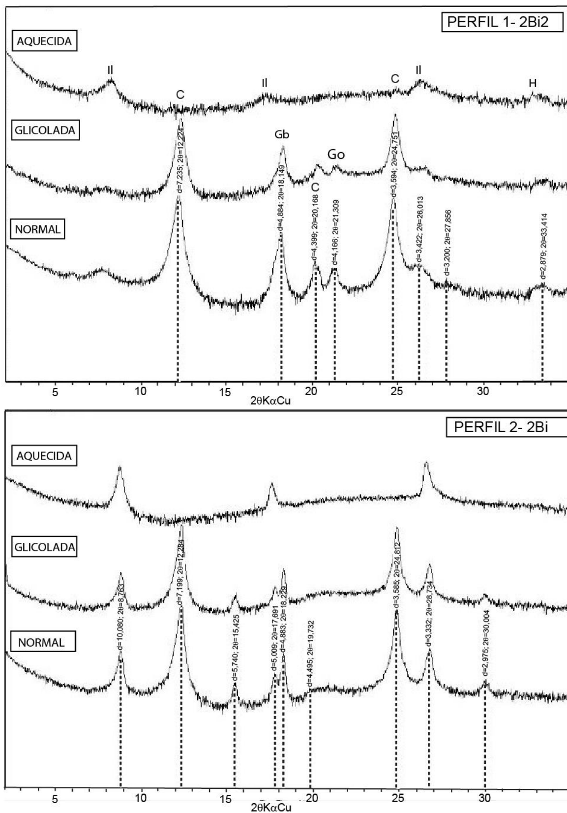
Figura 8: Difractogramas de Raios-X (° 2 Cu Kα) da fração argila < 2 μm secas ao ar, glicolada e aquecida (550°C) dos horizontes 2Bi2 e 2Bi, respectivamente dos perfis 1 e 2. C: caulinita; Gb: Gibbsita; Go: Goethita; H: Hematita; IL: Ilita.
