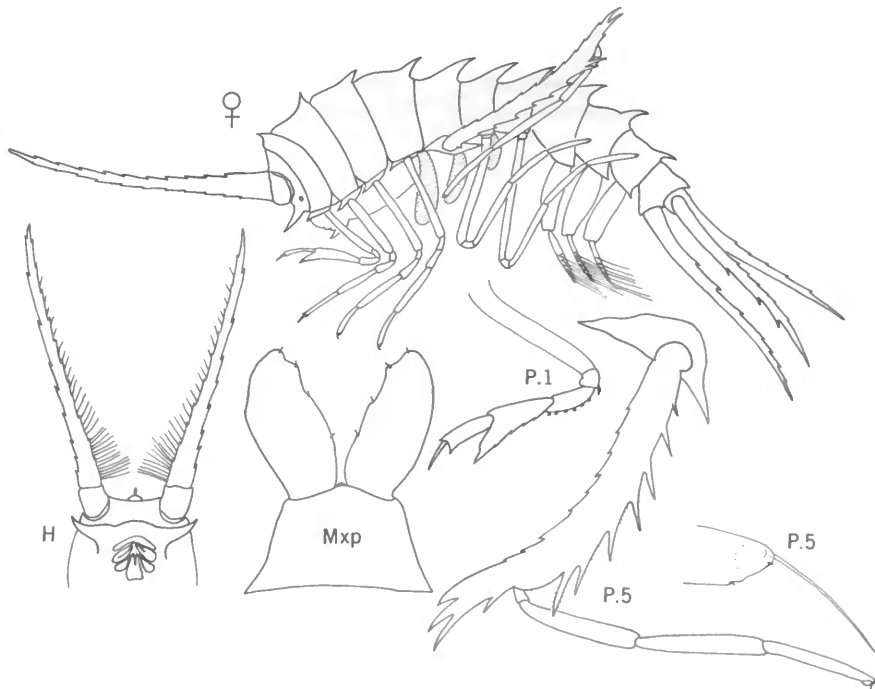
FIGURE 17.— Gtenoscina .
