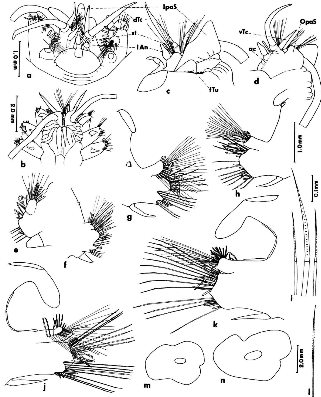
FIGURE 5.— Leanira robusta (syntype, USNM 10320): a , Anterior end, dorsal view; b , anterior end, ventral view; c , prostomium and left tentacular parapodium, inner or medial view; d , right tentacular parapodium, outer or lateral view; e , parapodium from segment 2, anterior view; f , parapodium from segment 3, posterior view; g , parapodium from anterior region, posterior view; h , same, anterior view; i , upper, middle, and lower neurosetae from same; j , parapodium from middle region, posterior view; k , same, anterior view; l , upper simple neuroseta from same; m , right seventh elytron; n , right middle elytron.
