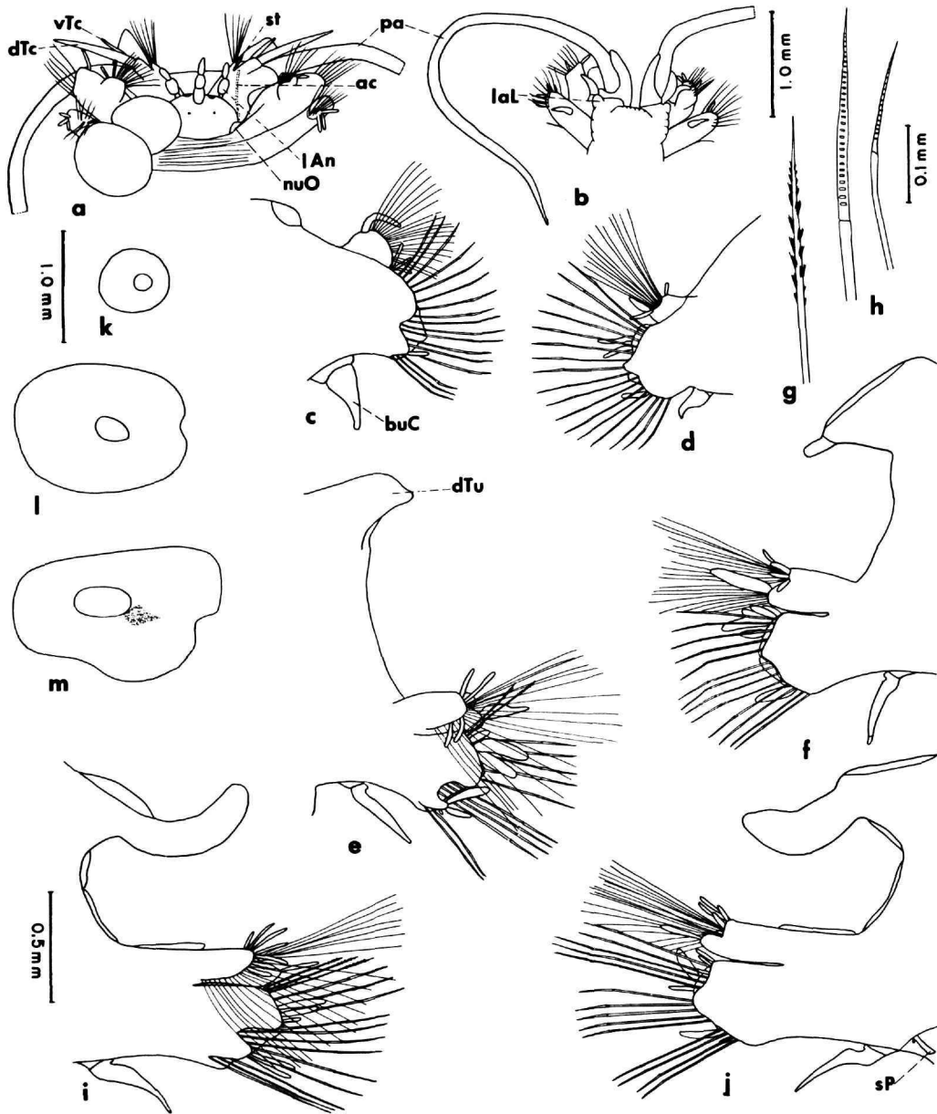
FIGURE 9.— Leanira adenensis , new species ( a, c-m , holotype, BMNH 1937: 9: 2: 61-62; b , paratype, USNM 40997): a , Anterior end, dorsal view, pharynx partially extended; b , same, ventral view; c , parapodium from segment 2, posterior view; d , parapodium from segment 3, anterior view; e , parapodium from anterior region, posterior view; f , same, anterior view; g , upper simple neuroseta from same; h , middle and lower compound neurosetae from same; i , parapodium from middle region, posterior view; j , same, anterior view; k , right first elytron; l , right elytron from anterior region; m , right elytron from middle region.
