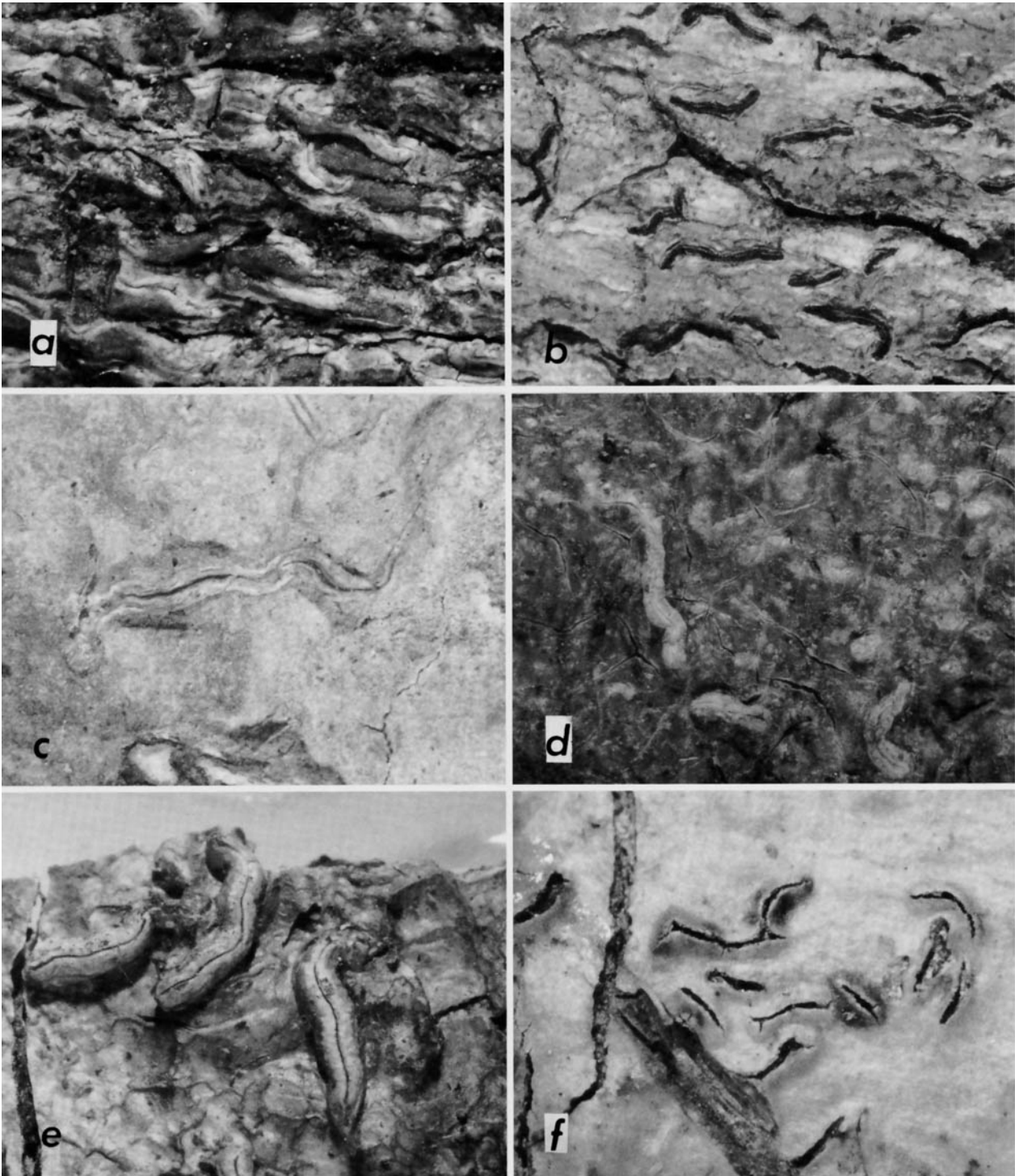
PLATE 8.—Species of Graphina : a, G. columbina (Wirth 446); b, G. dimidiata (Hale 35697); c, G. dispersa (Hale 38090); d, G. frumentaria (Hale 35242); e, G. illinata (Hale 35284); f, G. incrustans (Wirth 465).
