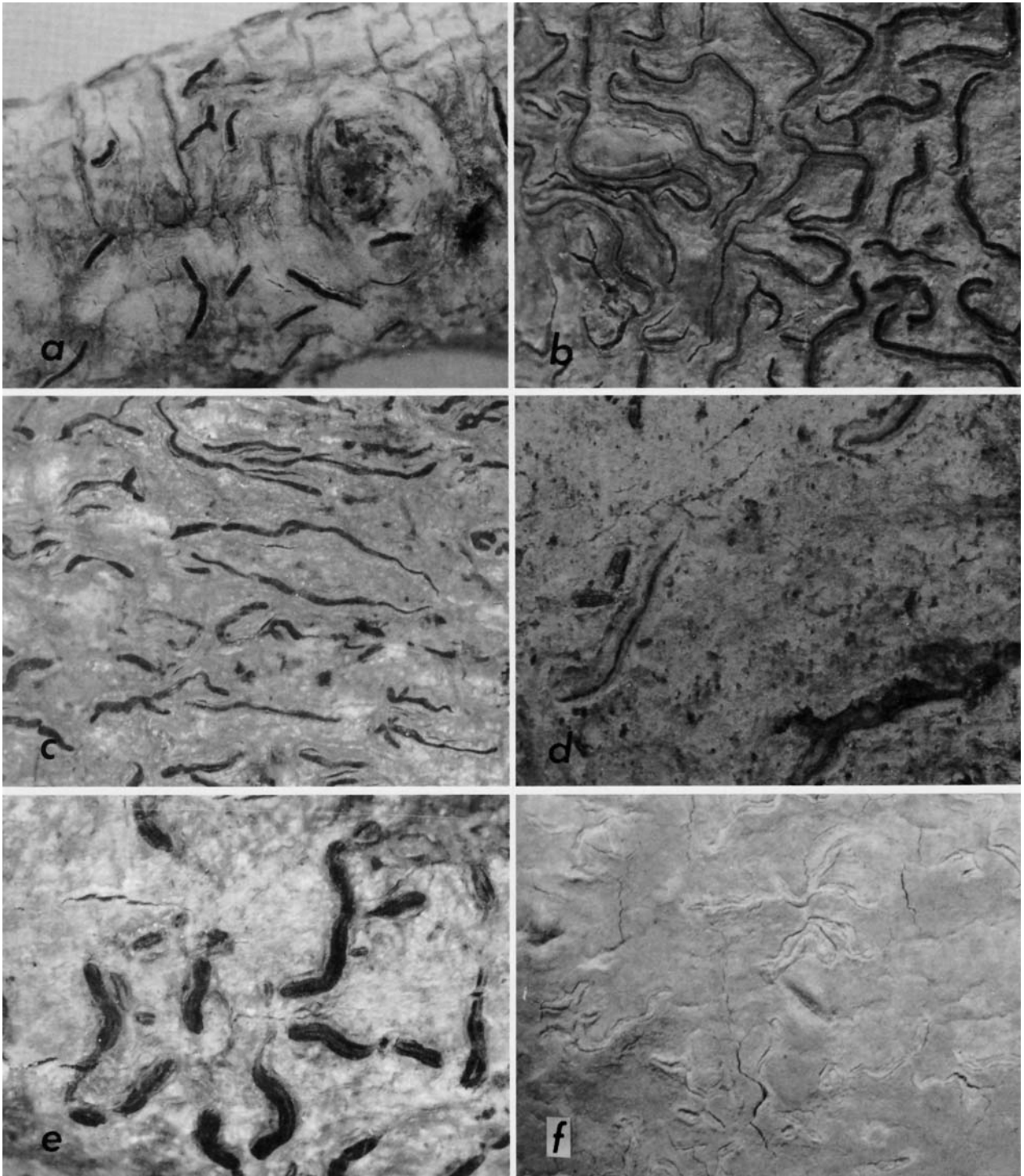
PLATE 10.—Species of Graphina : a, G. pseudoanaloga (Hale 35288); b, G. rufopallida (Elliott 1852); c, G. suberythrella (Imshaug 32699); d, G. triphoroides (Hale 35161); e, G. vestitoides (Imshaug 32859A); f, G. virginea (Wirth 547).
