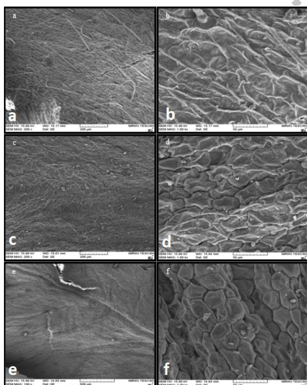
Fig. 2. SEM microphotographs of Trigonella L. leaves. a-b, T. filipes ; c-d, T. strangulata ; e-f, T. uncinata .
