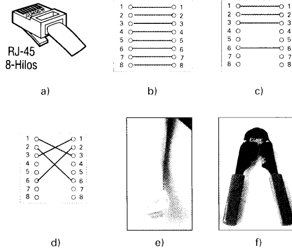
Figura 15.11. Conexiones en un conector RJ 45 para red Ethernet 10 Base T. a) Conector RJ 45; b) Cableado con conexión completa; c) Cableado con conexión mínima; d) Cableado para conectar dos ordenadores sin Hub; e) Aspecto de un cable crimpado al conector RJ 45; f) Alicates para crimpar.
