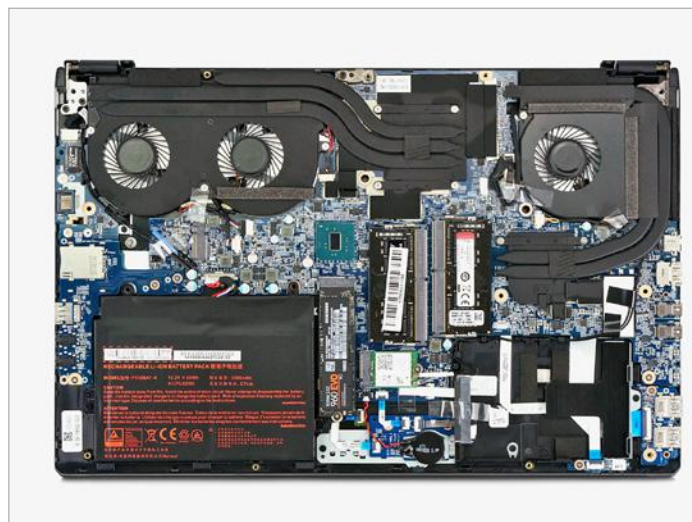
Die „Innereien“ eines Tuxedo Insanitybook: Während sich in älteren Modellen der Prozessor und die Grafikkarte die Heatpipes teilten, haben sie jetzt jeweils eigene.
