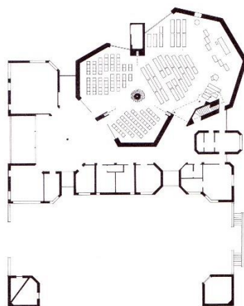
10. 1 Grundplan
