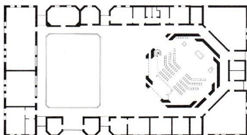
9. 1 Grundplan
