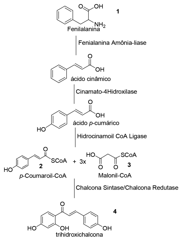
Figura 2. Rota biossintética de chalconas
