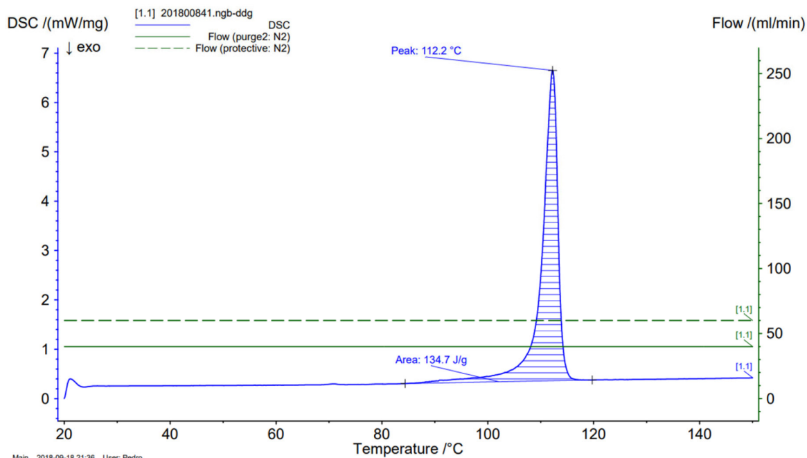
Figura 9. DSC da 1-(5-(2,6-difluorofenil)-4,5-di-hidro-3- p -tolilpirazol-1-il)etanona ( 9a )
