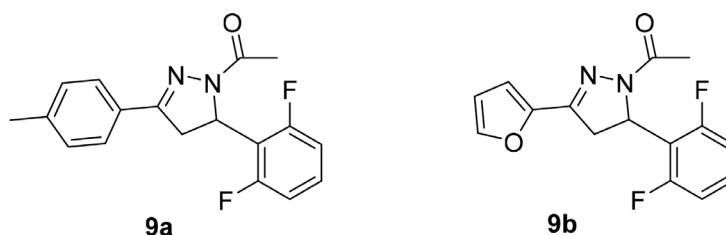
Figura 6. Estruturas dos compostos 9a e 9b
