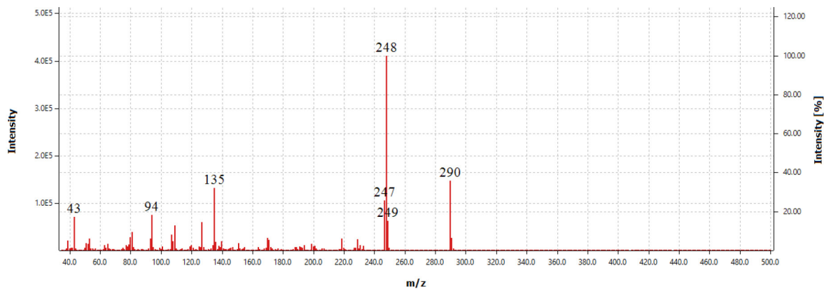
Figura 11. Espectro de massas da 1-(5-(2,6-difluorofenil)-3-(furan-2-il)-4,5-di-hidropirazol-1-il)etanona ( 9b )
