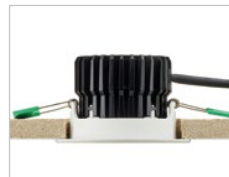
Einfache Montage durch das integrierte Betriebsgerät – nur 6,5 cm Einbautiefe notwendig
