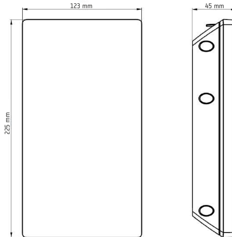
Abb. 1: Maße timeCard Terminal 3 mini
