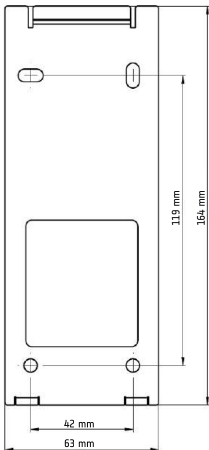
Abb. 2: Maße Wallbracket
