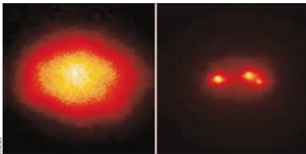
L'image d'une étoile triple prise sans optique adaptative (à gauche), puis avec ce procédé.
