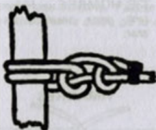
COTE DOBLE O VUELTA DE BRA- ZA.- Para amarrar una cuerda a un pos- te.
