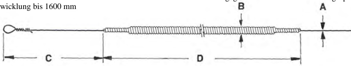
Handöse
