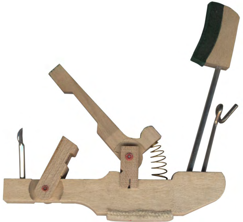
60041 Hebeglieder –Stück-
