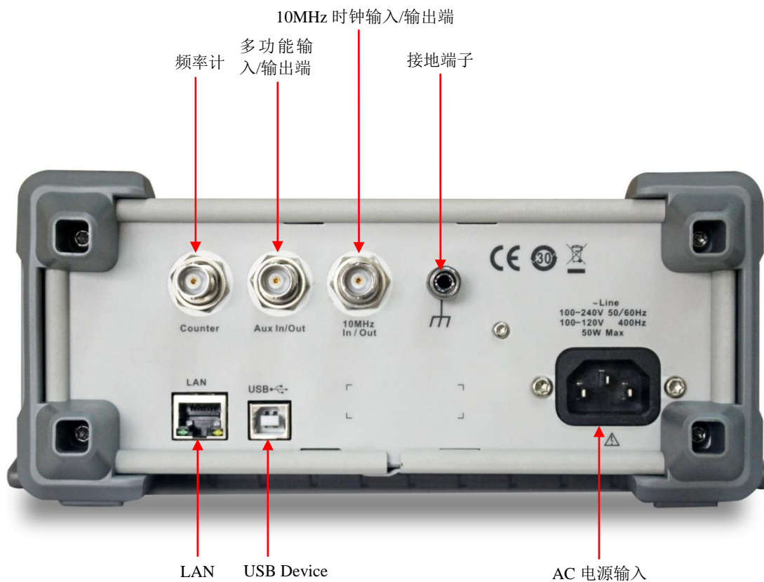
图 1-3 SDG1000X 后面板
