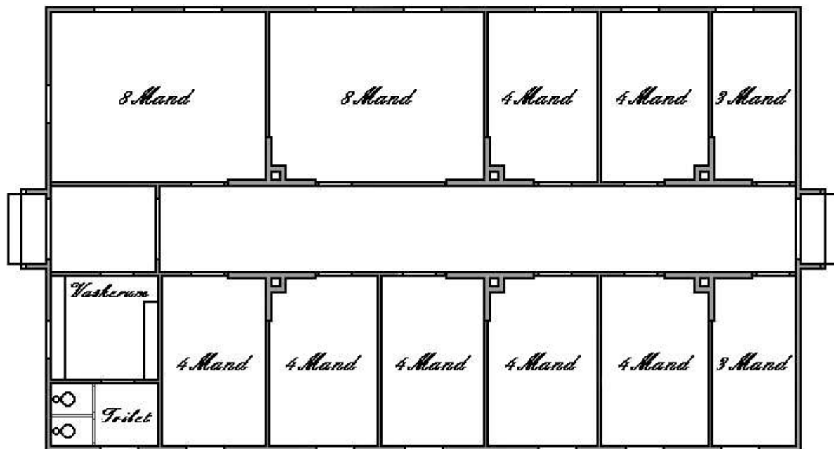
Plantegning af tysk 50 mands indkvarteringsbarak. De tyske barakker var inddelt i størrelserne: 10, 15, 25, 50, 100 og 120 mands barakker.
