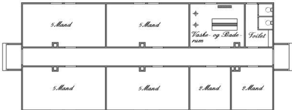
Plantegning af tysk 25 mands indkvarteringsbarak.
