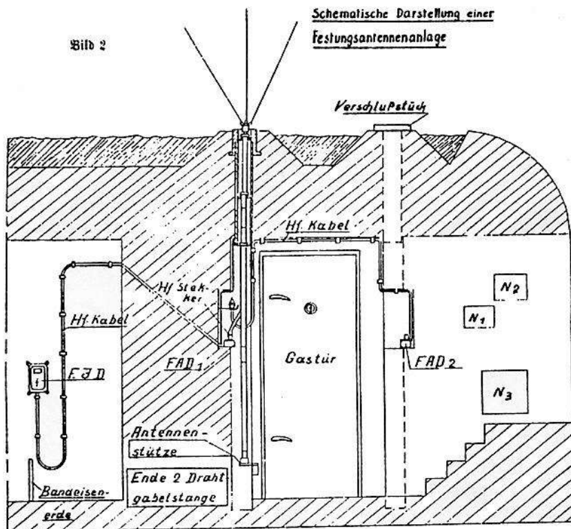
Fæstningsantennes placering i bunkerens indgangsparti.. Dok: SB
