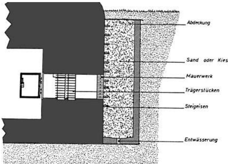
Nøddugang fra bunker. Dok. Peter Hansen
