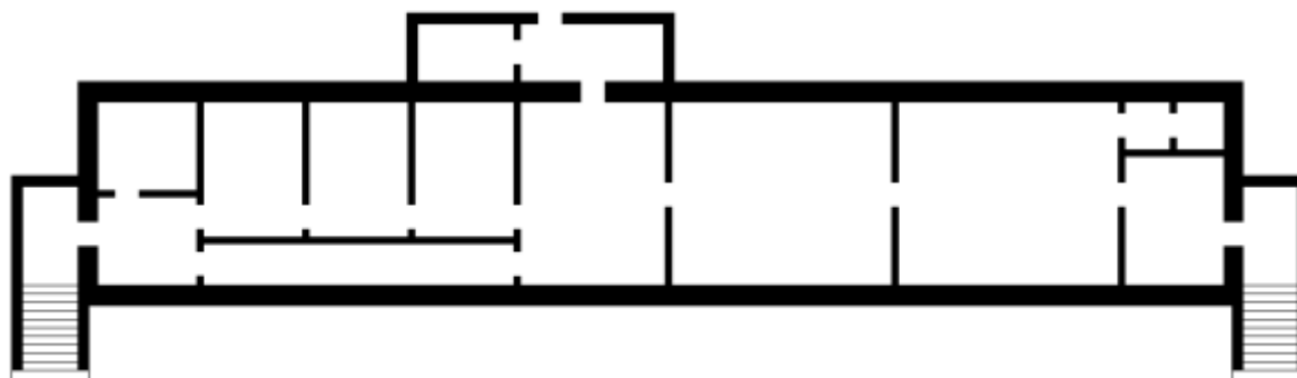
Tegning af infirmeri "bunker" under den tidligere Hjemmeværnsgård nord for flyvepladsen. Mål 47,0x9,5 m. Vægge og lofter 0,5 m. Teg: DM
