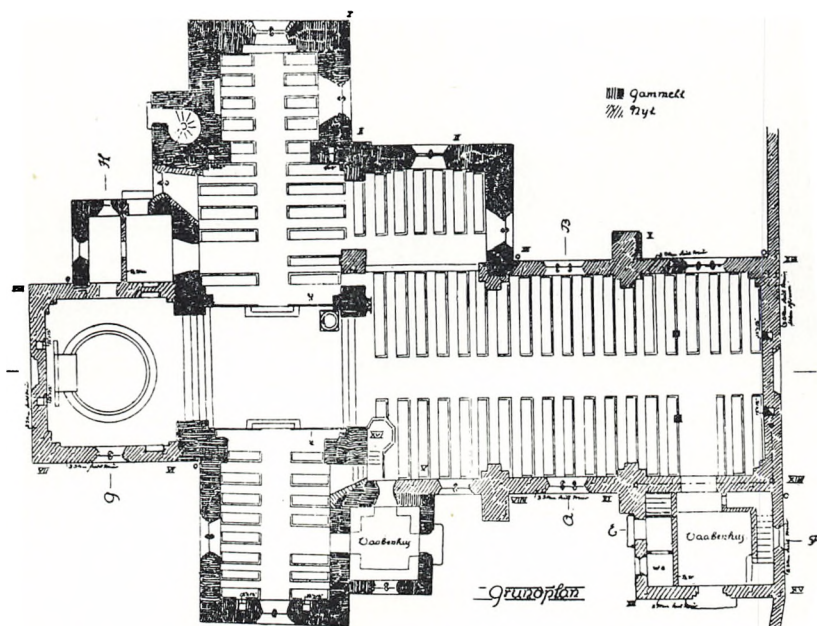
Arkitekt Lønborg-Jensens plan over kirkens ombygning 1914-16.
