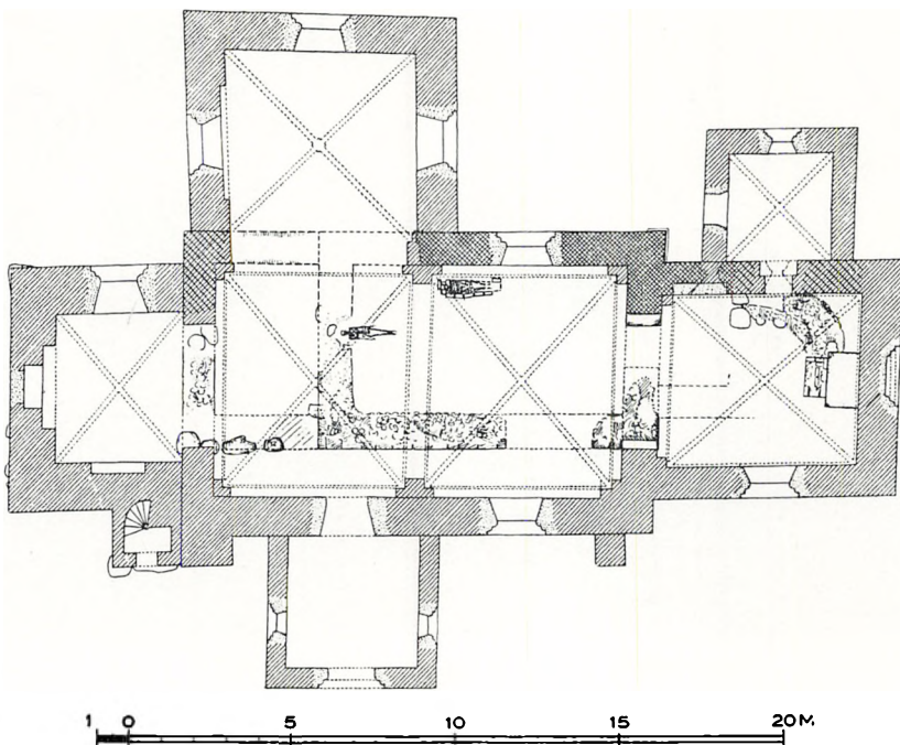
Haslev før Ombygningen 1914—16. Plan. 1 : 300. Tegnet af C. G. Schultz 1936 paa Grundlag af Th. Havnings, M. Clemmensens og C. A. Jensens Opmaalinge.
