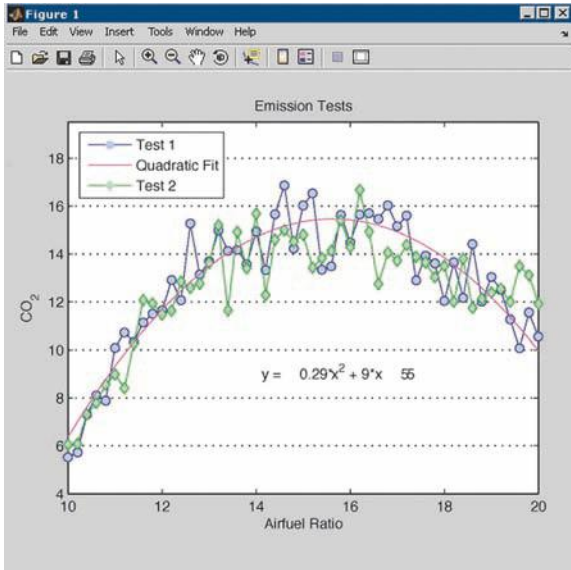
Рис. 2. Аппроксимация зависимости уровня эмиссии ДВС, построенная на реальных данных
