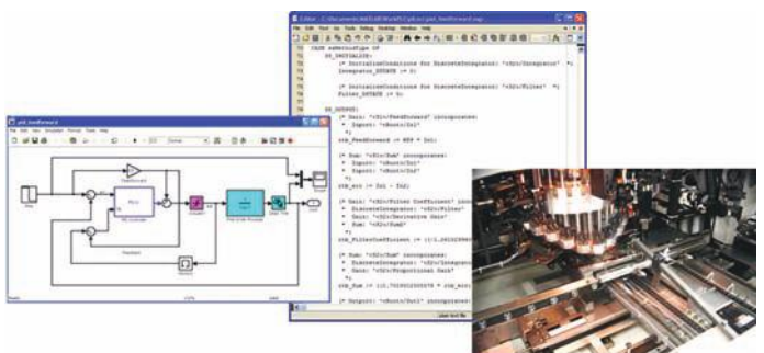
Работа в Simulink PLC Coder: автоматически генерируемый код — быстрый шаг от построения модели к готовой промышленной системе управления.
