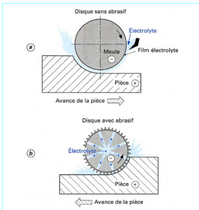
Figure 16 – Rectification électrochimique
