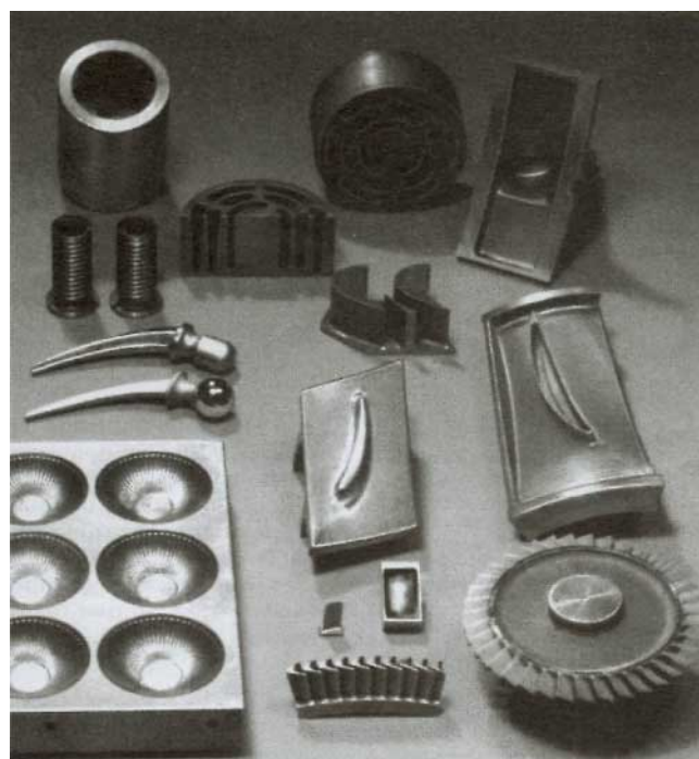
Figure 20 – Exemples de pièces usinées par ECM (doc. AEG-Elotherm)
