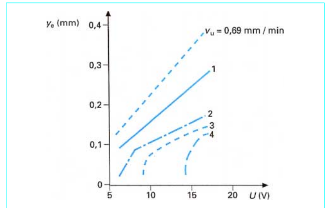
Figure 7 – Variation du gap en fonction de la tension d’alimentation pour une vitesse d’avance donnée
