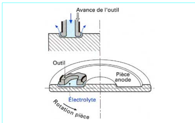
Figure 17 – Tournage électrochimique
