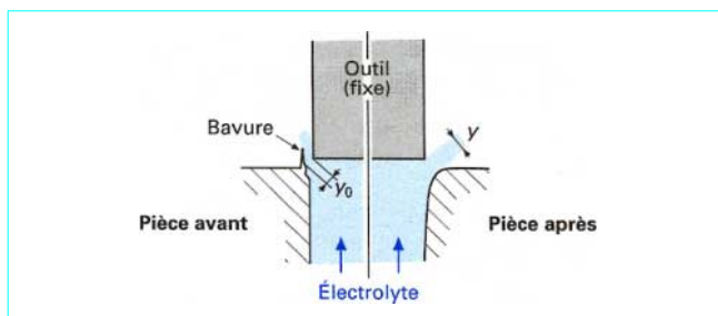
Figure 15 – Usinage statique : exemple de l'ébavurage
