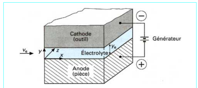
Figure 3 – Gap entre électrodes planes parallèles avec une tension constante
