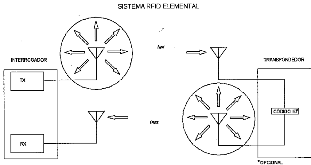
Fig. 1.2 Esquema de un sistema RFID elemental.
