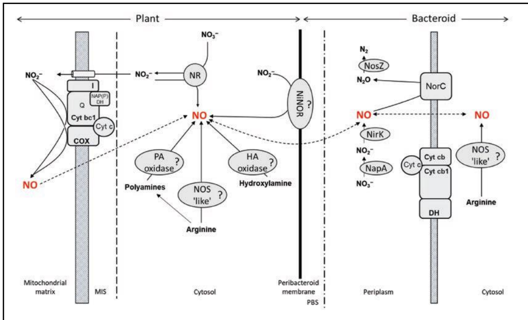
Figure 21 : Synthèse du NO lors de la symbiose.
