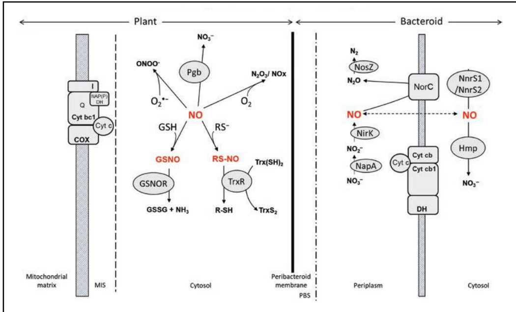
Figure 22 : Dégradation du NO lors de la symbiose.
