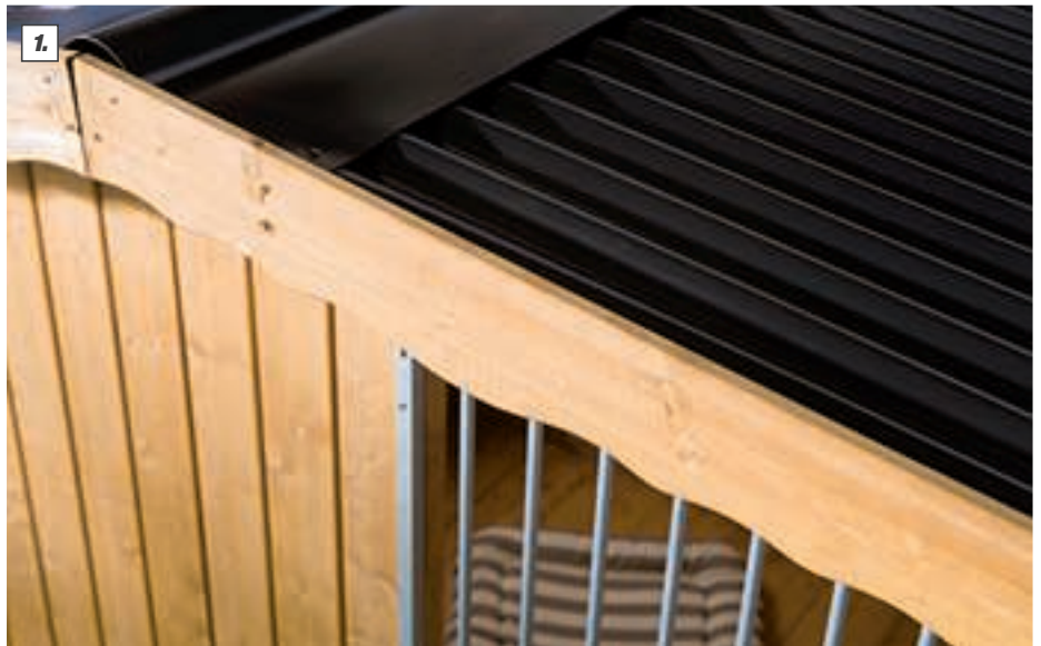
1. „SALUX WBS“ PVC-Wellplatte * Als Ersatz bzw. Alternative von/zu Bitumenplatten bestens geeignet. 2.000 x 900 x 1,2 mm (L x B x S)
