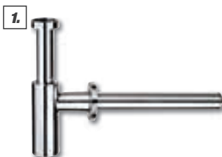
1. Design-Tassen-Geruchsverschluss 1 1/4" Ø 32 mm mit Tauch- und Wandrohr, inkl. Rosette, Messing, verchromt, Art.-Nr. 5467539 39.99
