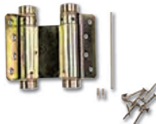
11. Pendeltürbänder 75 x 110 vz Mit Stellstift und Stellniet, gelb-verzinkt. Maße: 75 x 110 mm (L x H). Art.-Nr. 1727385
