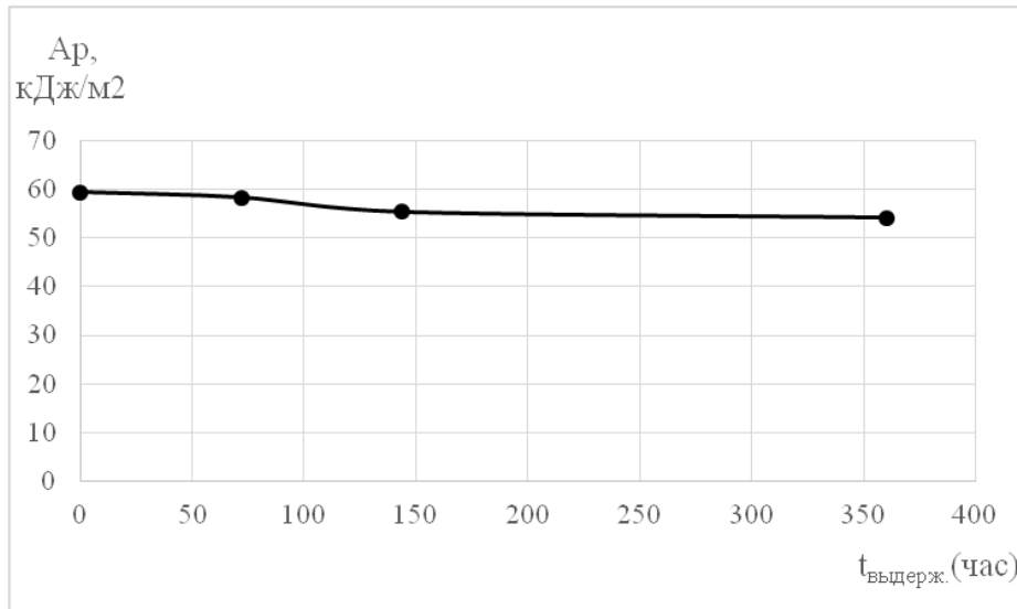
Рис. 5 График зависимости затрачиваемой энергии на единицу площади поперечного сечения полимерного образца для деформации (разрушения) от времени пребывания образца в печи термостарения для ПКМ из ПА-6 с 5% содержанием наполнителя
