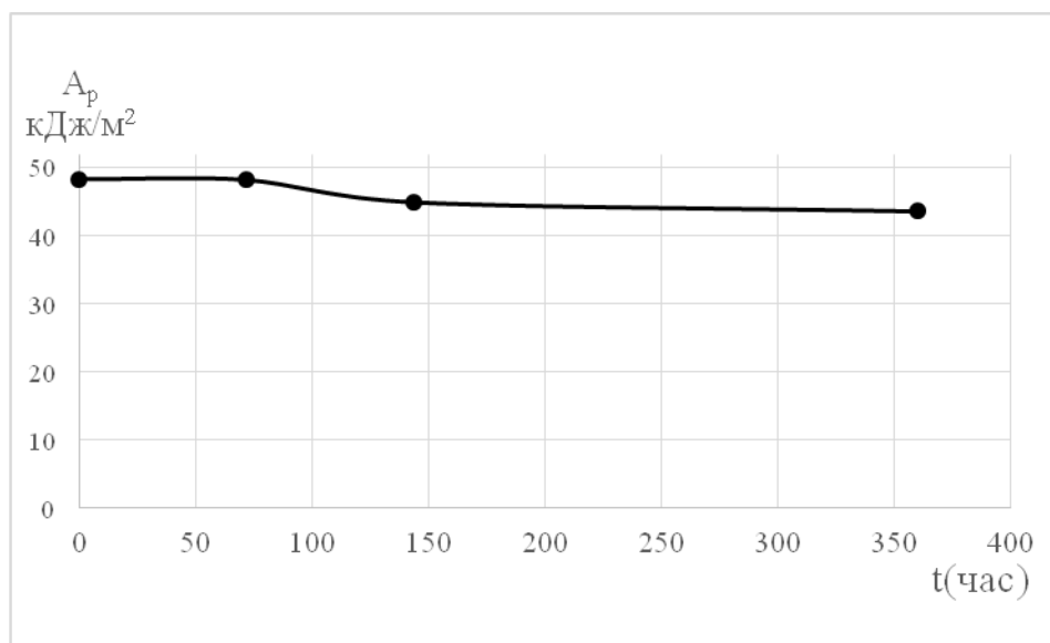
Рис. 1 График зависимости затрачиваемой энергии на единицу площади поперечного сечения полимерного образца для деформации (разрушения) от времени пребывания образца в печи термостарения для ПКМ из ПА-6 без стабилизирующих добавок
