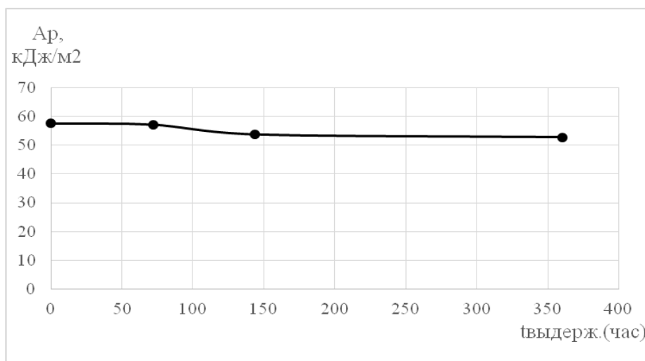
Рис. 3 График зависимости затрачиваемой энергии на единицу площади поперечного сечения полимерного образца для деформации (разрушения) от времени пребывания образца в печи термостарения для ПКМ из ПА-6 с 1.5% содержанием наполнителя
