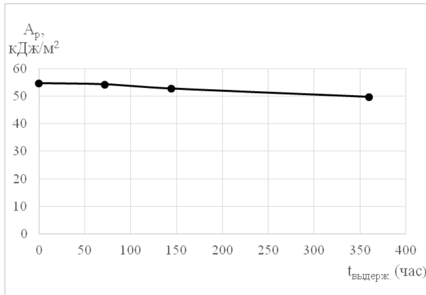
Рис. 2 График зависимости затрачиваемой энергии на единицу площади поперечного сечения полимерного образца для деформации (разрушения) от времени пребывания образца в печи термостарения для ПКМ из ПА-6 с 0.5% содержанием наполнителя
