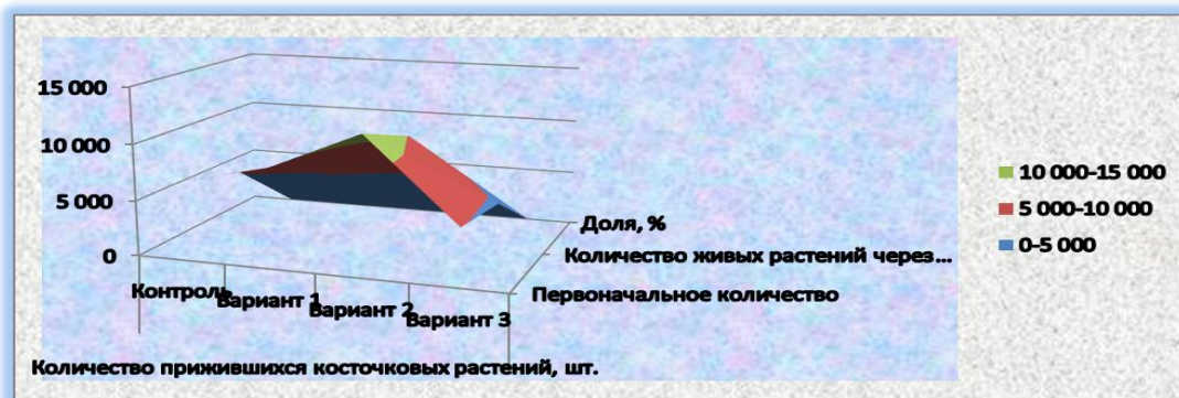
Рис. 3. Приживаемость микрорастений косточковых подвоев и сортов (2011-2020 гг.)
