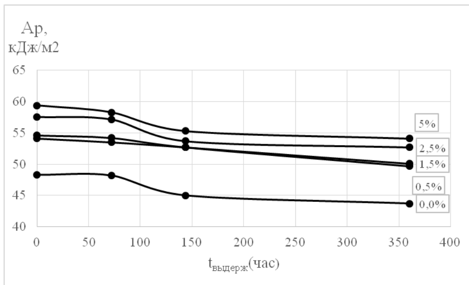
Рис. 6 Обобщенный график для сравнения полученных результатов по прочности ПКМ с различной концентрацией стабилизирующего наполнителя.
