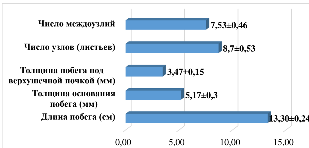
Диаграмма 2. Средние морфометрические показатели однолетних побегов Castanea sativa
