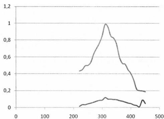
Рисунок 4. Результаты анализа электронных спектров поглощения спиртового раствора растительного сырья и стандартного раствора олеаноловой кислоты.
