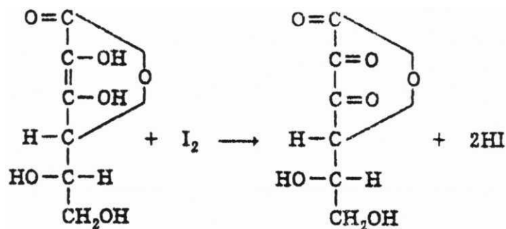
Рисунок №2. Титрование йодометрическим методом.
