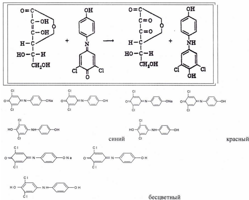
Рисунок №1. Титрование раствора 2,6-дихлорфенолиндофенолятом натрия.
