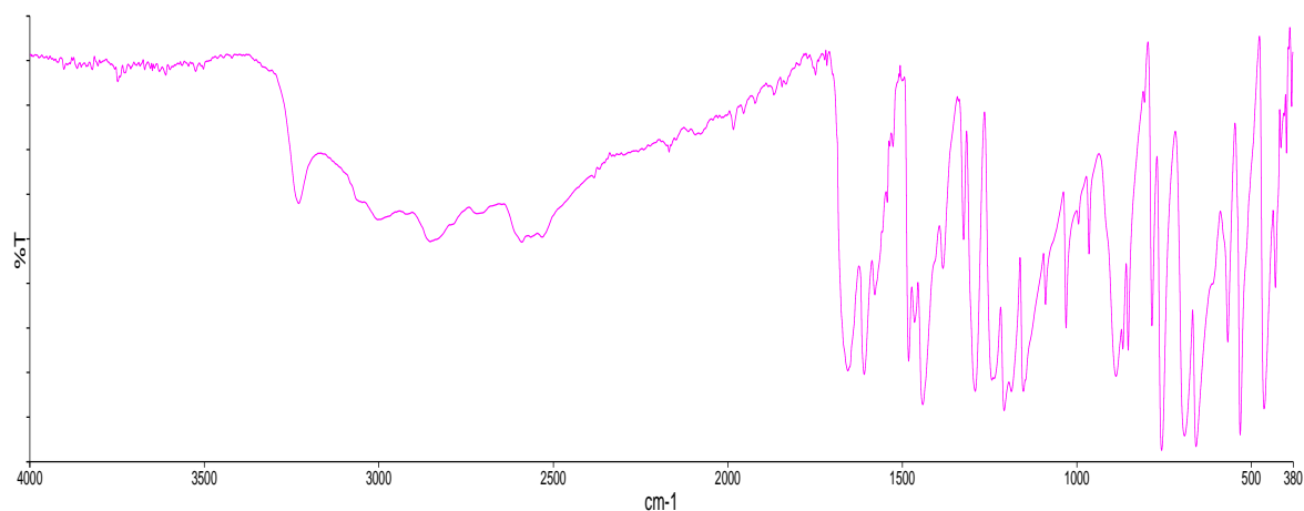
Рисунок 1. ИК-спектр салициловой кислоты
