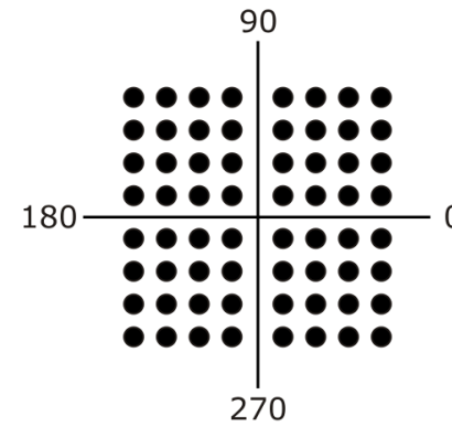
QAM-64 6 bits por símbolo
