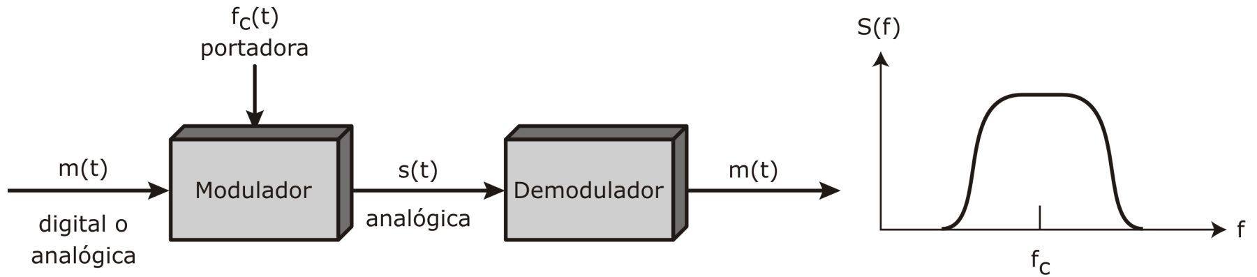
Modulación en una señal analógica
