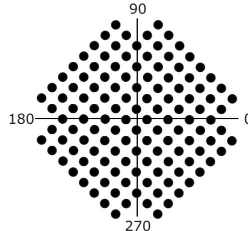
V32 bis (14400 bps)
