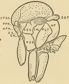
17. POLYLEPTA
