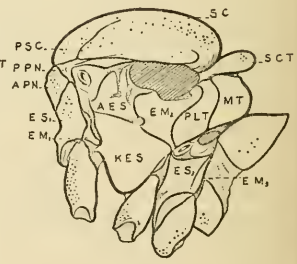
45. PSEUDOSCIARA
