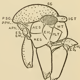
27. CYCLONEURA
