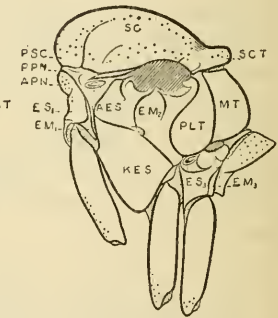
44 SCIARA
