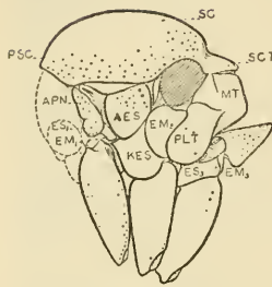
37 CORDYLA
