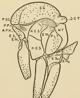
24. BOLETINA
