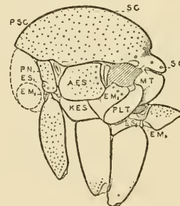
42. EPICYPTA
