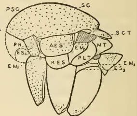
43. SCEPTONIA
