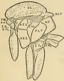
10. PLATYURA
