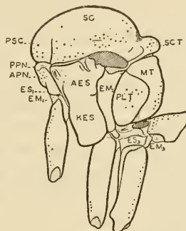
22. SCIOPHILA
