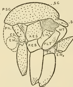
41. OPISTHOLOBA
