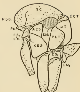
25. DZIEDZICKIA
