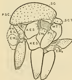
39 MYCETOPHILA
