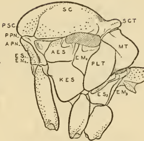
13 FENDEROMYIA
