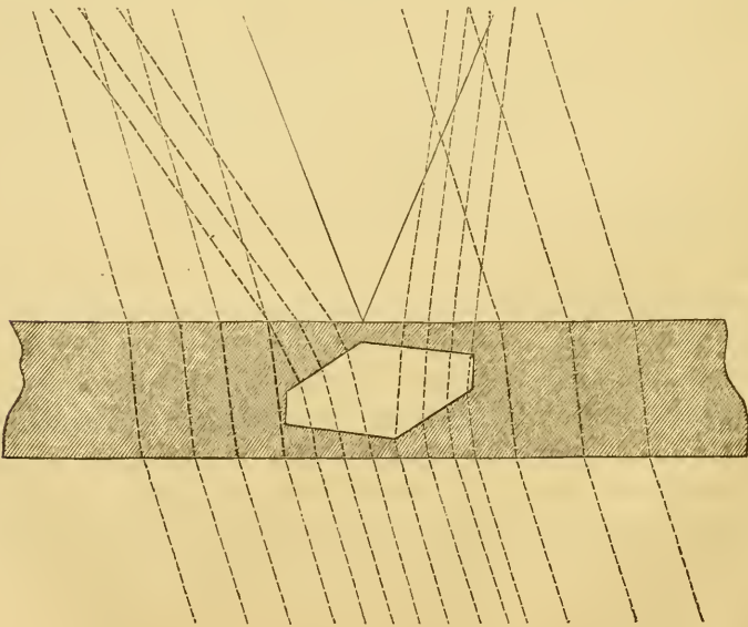
Corte del cristal de augita con la cavidad, normalmente á las caras de la preparación Porfirita augítica del Puente de Segovia.
