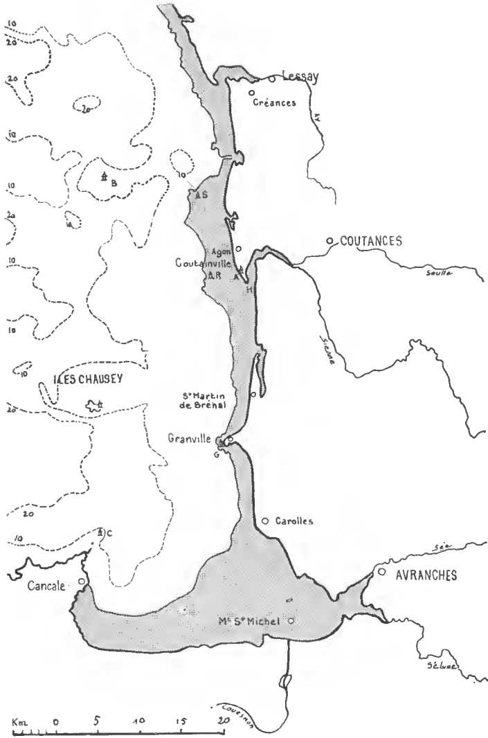
FIG. 1. — Carte de la côte ouest du Cotentin, du Mont Saint-Michel au hâvre de Lessay. Échelle : 1/625.000. En grisé, zone des plus basses mers de vives-eaux.
