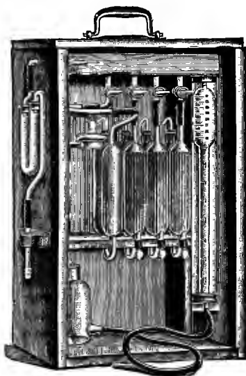
FIG. 154.—Orsat-Lunge gas analysis apparatus.
