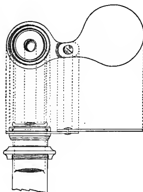
FIG. 49.—Eye shade.
