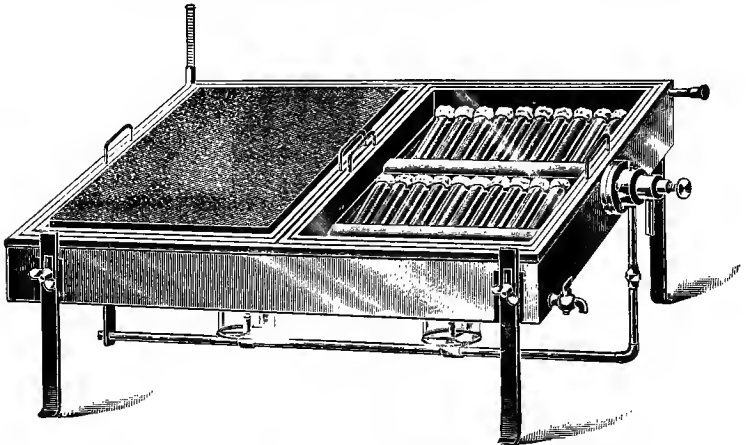
FIG. 110.—Serum inspissator.
