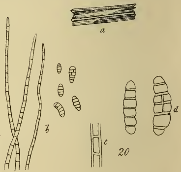
Helminthosporium delicatulum.
