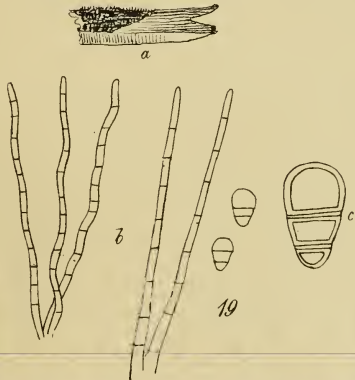
Helminthosporium obovatum.
