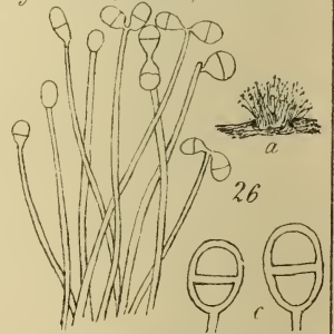
Dactylum obovatum.
