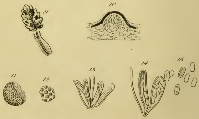
Sphaeria Rhytismoides.
