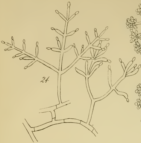
Botrytis terrestris.
