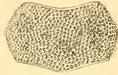
Fig. 7. — T. cribricollis , n. sp. Pronotum.
