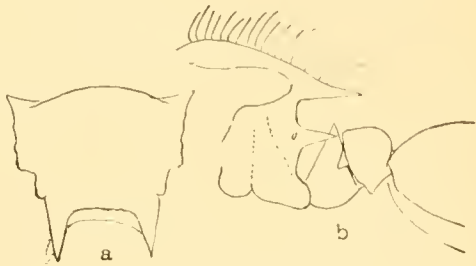
Fig. 4. — Meranoplus Bondroiti , n. sp. a , thorax vu de dessus (en pointillé les épines épino-tales); b , profil du thorax et du pédicule.
