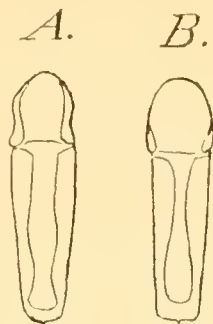
Fig. 5. — Pénis, A, de Thyamis onosmatis Peyerh. — B, de T. multipunctata All.
