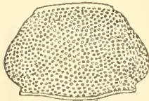
Fig. 1. — N. borbonica , n. sp. Pronotum.
