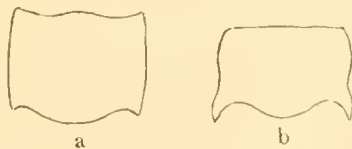
Fig. 2. — Phyracaces Foreli Santschi. Pédicule a ♀, b ♂.
