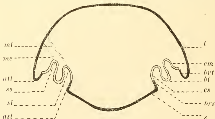
Fig. 1. — Schéma de la coupe transversale d'un segment pré-génital chez les Phasmides (exosquelette en traits pleins, muscles respiratoires en pointillé).
