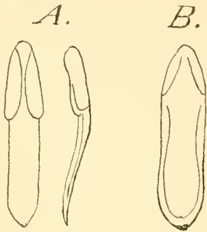
Fig. 4. — Pénis. A, d' Aphthona Beauprei Pic. — B, d' A. Perrisi silvana , n. subsp.
