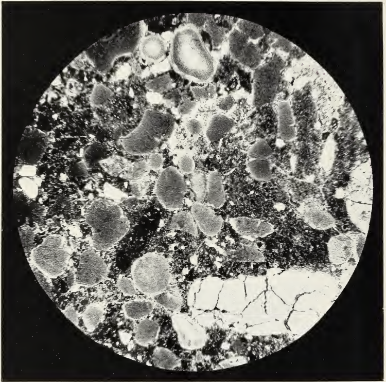
Aspect général des grains de Glaucopine dans un nodule phosphaté.
