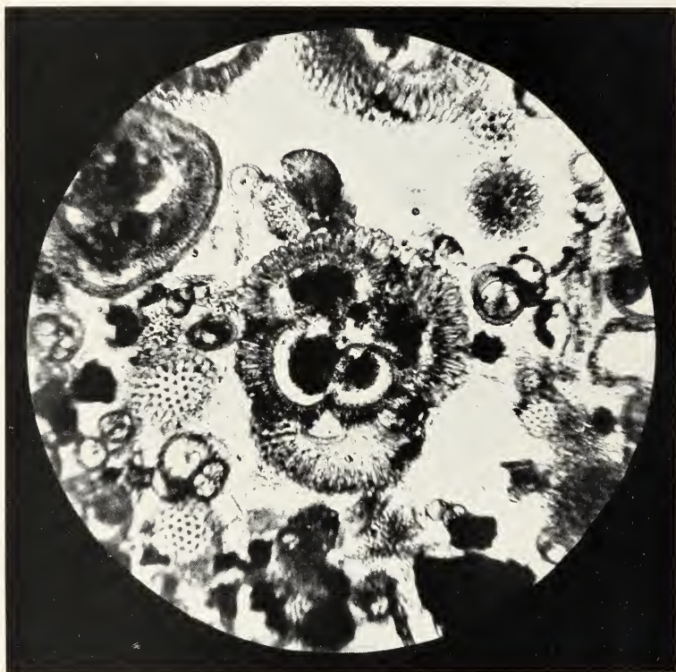
Boue à Globigérines provenant de la Station 176 ( Challenger ). La coquille occupant le centre de la figure est en partie remplie par une matière argileuse brune, et constitue un moule imparfait.
