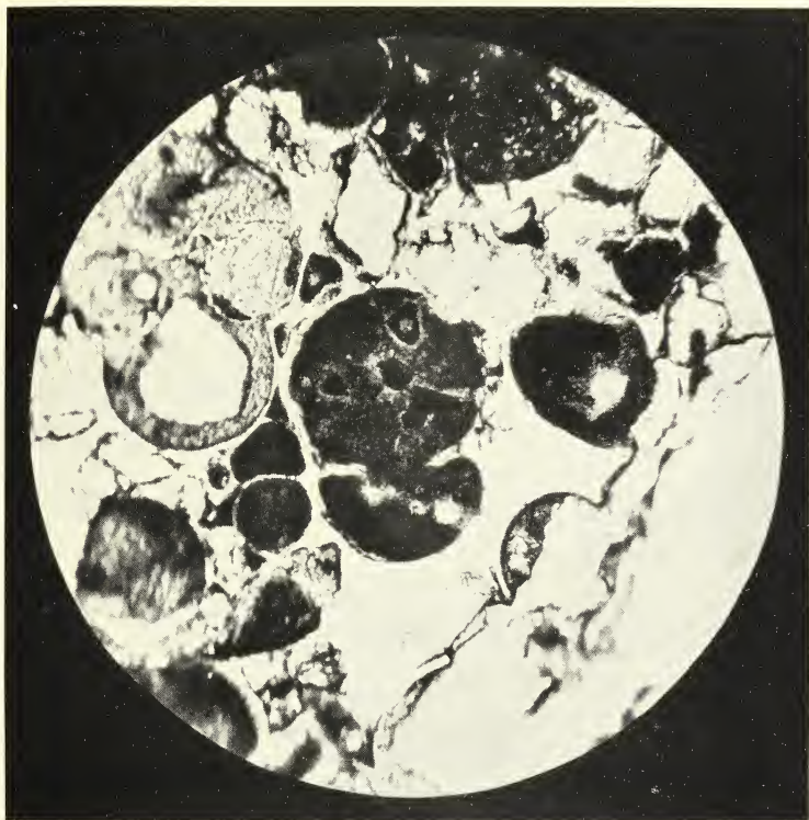
Sable vert recueilli par le Challenger à la Station 154 par 750 m. Le centre de la figure est occupé par un moule glauconitique contenant des inclusions opaques.
