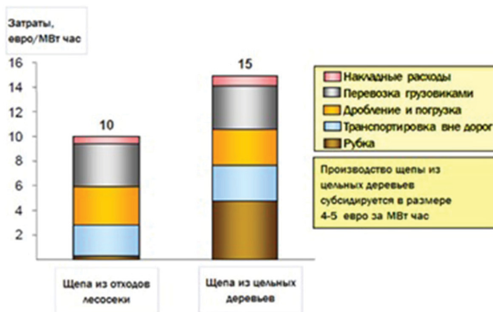
Рис. 3. Структура себестоимости производства щепы в Финляндии
