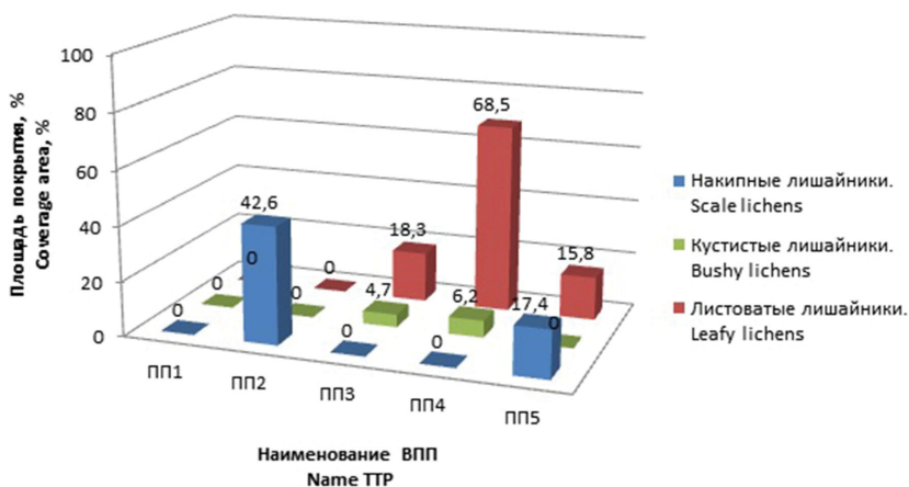
Рис. 4. Площадь покрытия ствола дерева лишайниками на высоте до 1 м (трансекта на север) Fig. 4. The area of the tree trunk with lichens at a height up to 1 meter (transsect to the north)
