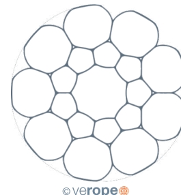
Abb. 8: Unverdichtete und verdichtete Rundlitzen
