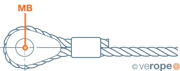
Vollkausche verpresst
