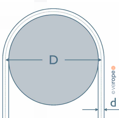
Abb. 73: Scheibendurchmesser
