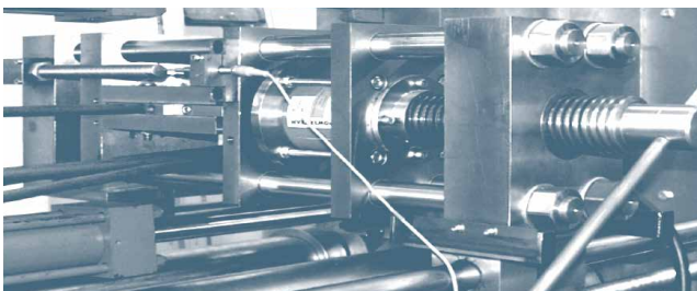
Abb. 62: Prüfprinzip zur Messung des Querelastizitätsmoduls unter Zugkraft (Quelle: TU Clausthal)
