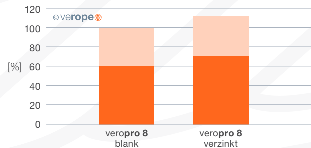
Abb. 50: Biegewechselvergleich von blanken und verzinkten Seilen
