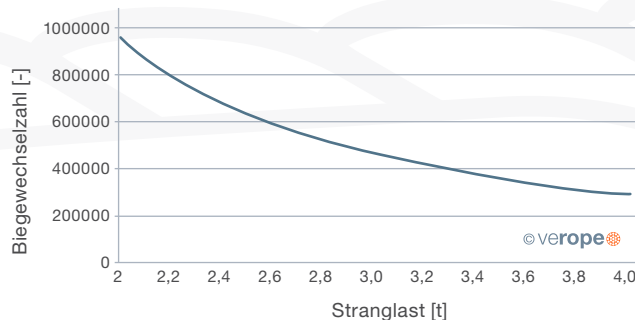
Abb. 52: Einfluss der Stranglast auf die Seillebensdauer
