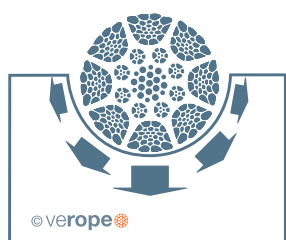
veropower 8 mit verdichteten & gehämmerten Außenlitzen
