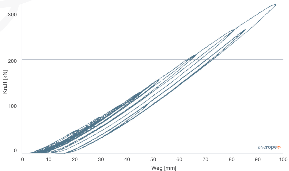
Abb. 54: Kraft-Wegdiagramm eines verope® Spezialdrahtseiles zur Bestimmung des Elastizitätsmodul
