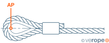
Kausche verpresst
