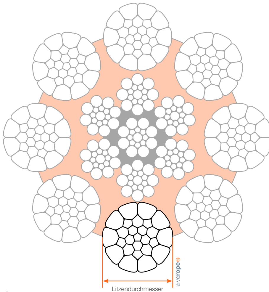
Abb. 4: Litzendurchmesser
