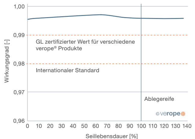
Abb. 71: Wirkungsgradmessung über der Seillebensdauer unter Belastung
