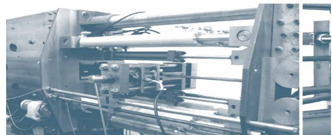
Abb. 62: Prüfprinzip zur Messung des Querelastizitätsmoduls unter Zugkraft (Quelle: TU Clausthal)
