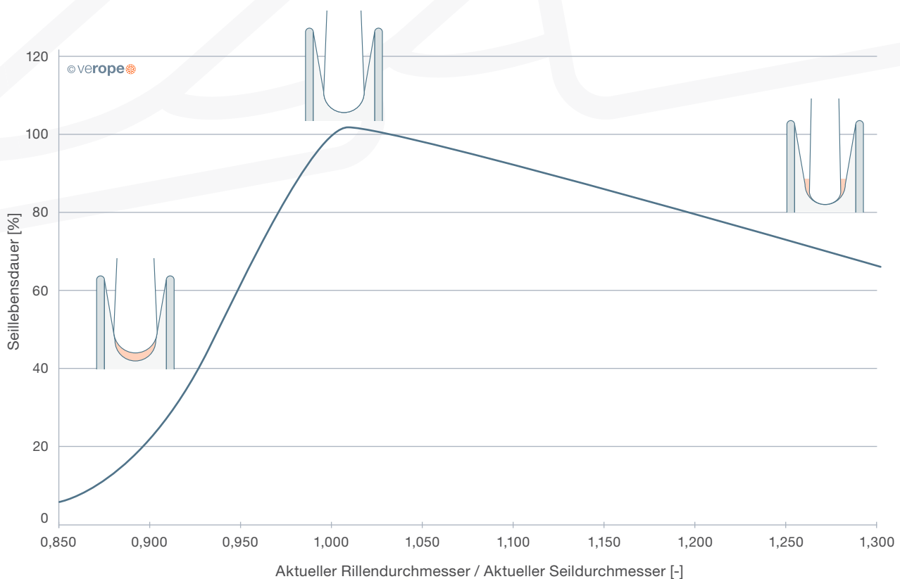
Abb. 51: Einfluss des Rillendurchmessers auf die Seillebensdauer (siehe auch Seite 60)
