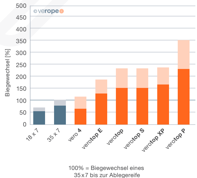
Abb. 48: Biegewechsel drehungsfreie Seile unter gleicher Belastung bis zur Ablegereife und bis zum Bruch
