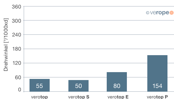
Abb. 66: Drehwinkel unter einer Belastung von 20% der Mindestbruchkraft
