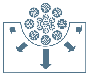
veropro 8 mit verdichteten Außenlitzen
