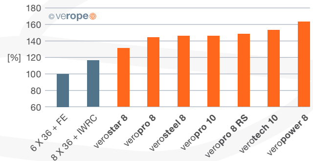
Abb. 30: Bruchkräfte nicht drehungsfreier Seile
