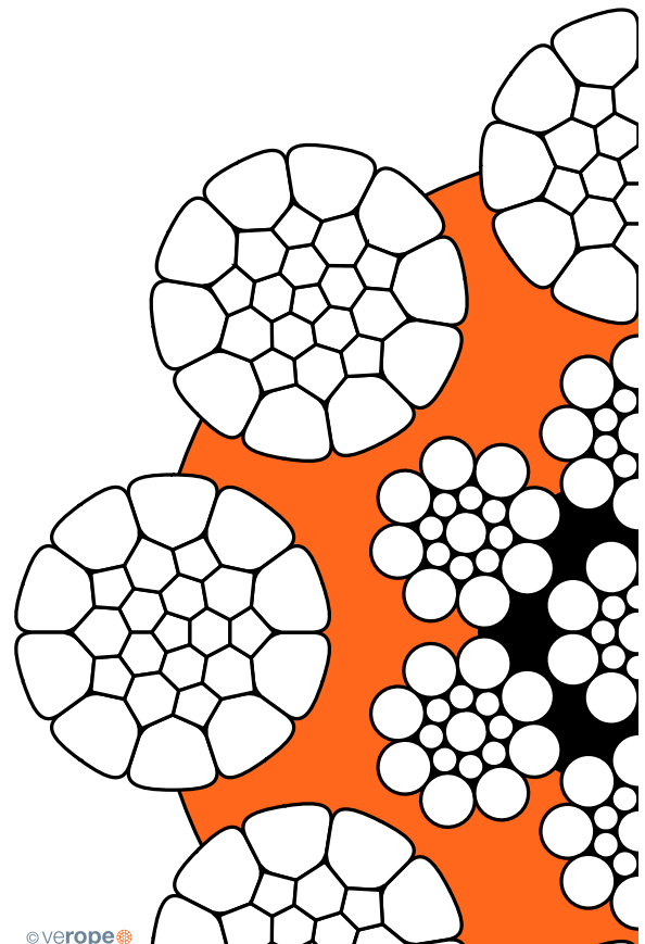
Abb. 29: Die Kunststoffzwischenlage (orange dargestellt)
