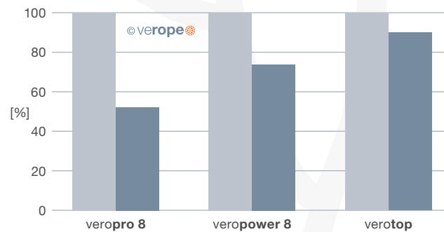
Abb. 32: Bruchkräfte eines neuen Seiles im Zerreißversuch ohne und mit Wirbel
