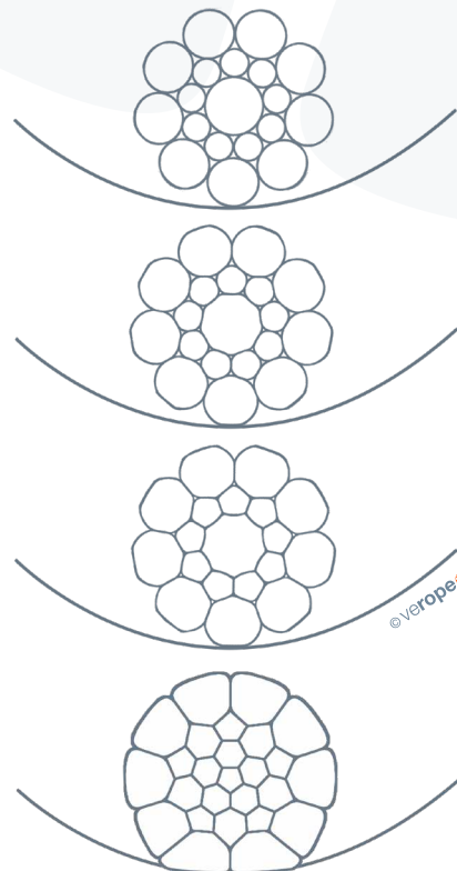
Abb. 24b: Litzenauflage
