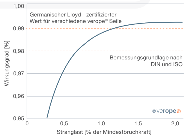
Abb. 69: Wirkungsgradmessung im niedrigen Lastbereich bis 2 % der Mindestbruchkraft
