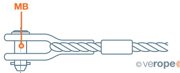
Gabelkausche verpresst
