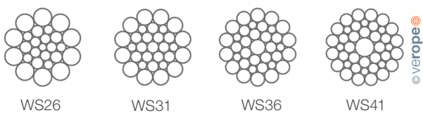
Abb. 7: Litzenmacharten
