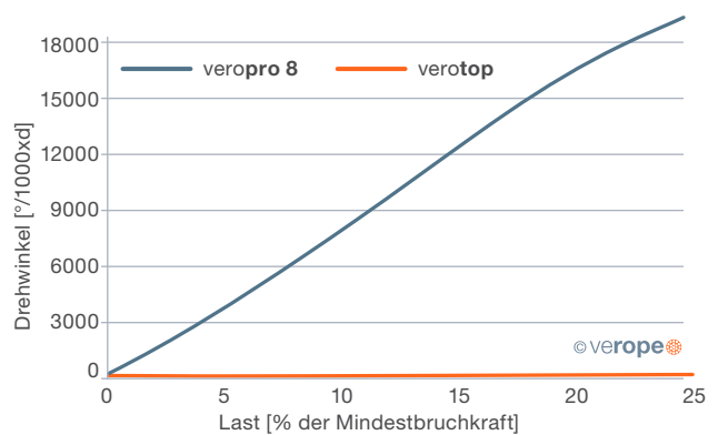
Abb. 64: Drehwinkelversuch veropro 8 und verotop
