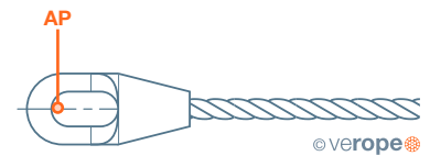
Bügelseilhülse: Metall- oder Kunstharzverguss
