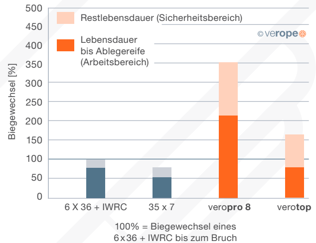
Abb. 46: Zahl der Biegewechsel bis zur Ablegereife und bis zum Bruch
