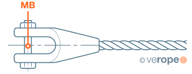
Gabelseilhülse: Metall- oder Kunstharzverguss
