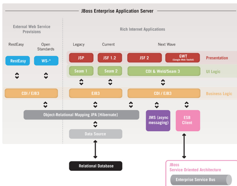
Obr. 6-11: Architektura aplikačního serveru (Zdroj: http://www.advancedcomputersoftware.com )
