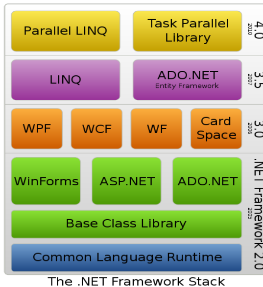
Obr. 5-1: Architektura .NET frameworku (zdroj: http://en.wikipedia.org/wiki/File:DotNet.svg )
