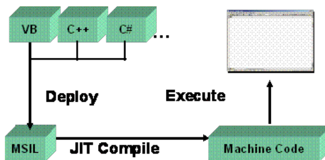
Obr. 5-2: Princip kompilace a spuštění .NET aplikace
