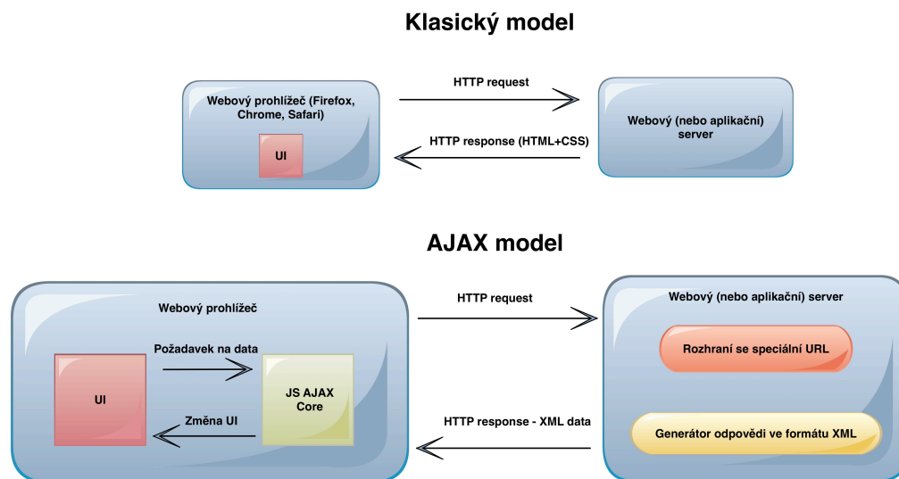
Obr. 8-1: Základní schéma architektury technologie AJAX
