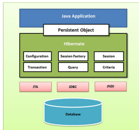
Obr. 6-22: Architektura Hibernate (Zdroj: http://www.tutorialspoint.com )
