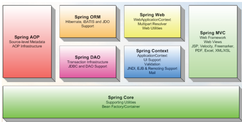
Obr. 6-25: Spring a jeho součásti (Zdroj: http://www.developersbook.com )
