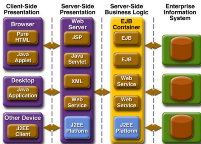
Obr. 6-10: Java EE komponenty v logických vrstvách aplikací (Zdroj: Suresh Devang)
