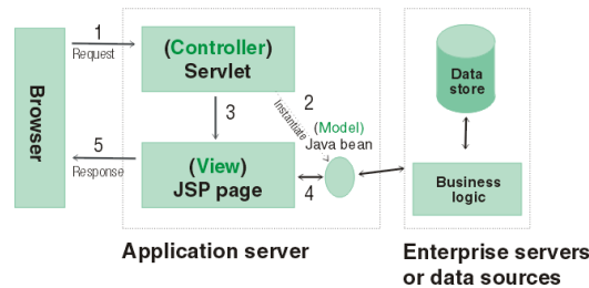
Obr. 6-14: Architektura JSP (Zdroj: IBM)
