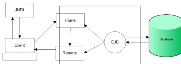
Obr. 6-18: Architektura EJB (Zdroj: http://sanjaal.com )
