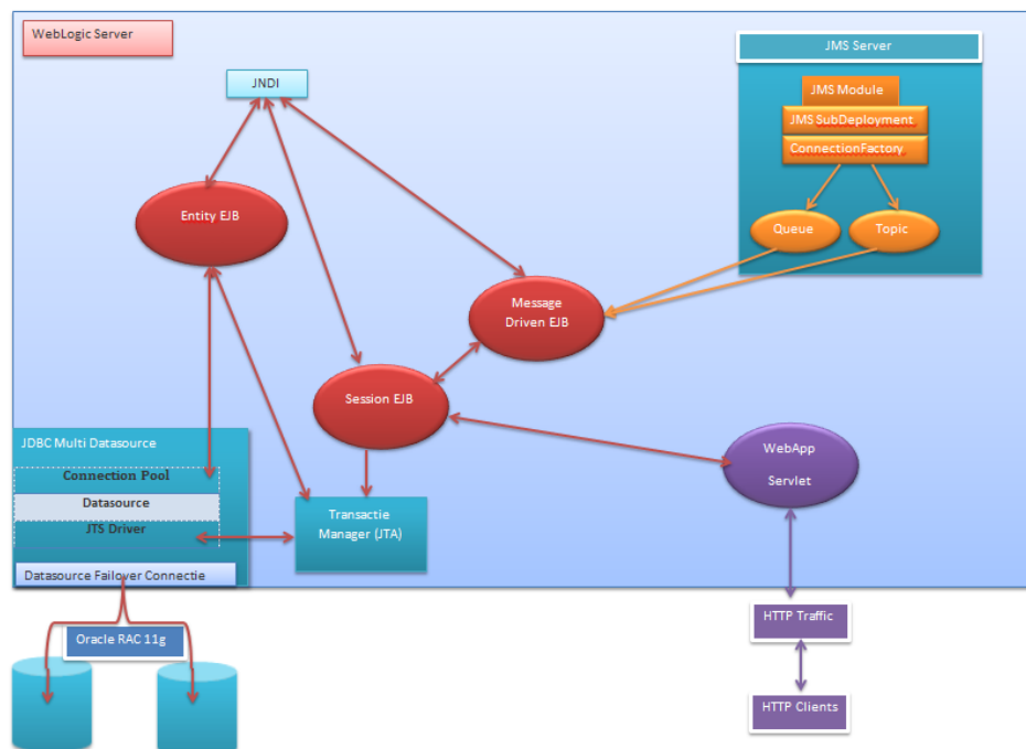
Obr. 6-19: Architektura EJB začleněná do AS Weblogic (Zdroj: http://technology.amis.nl )
