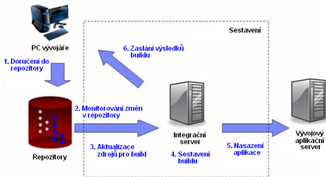
Obr. 1-12: Postup a struktura neustálé integrace
