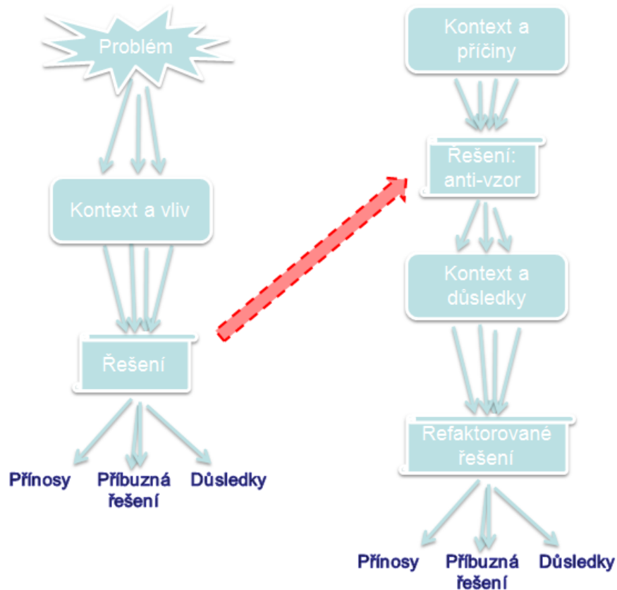
Obr. 10-1: Koncept vzorů a anti-vzorů (struktura a smysl jednotlivých částí), zdroj: [AP1]
