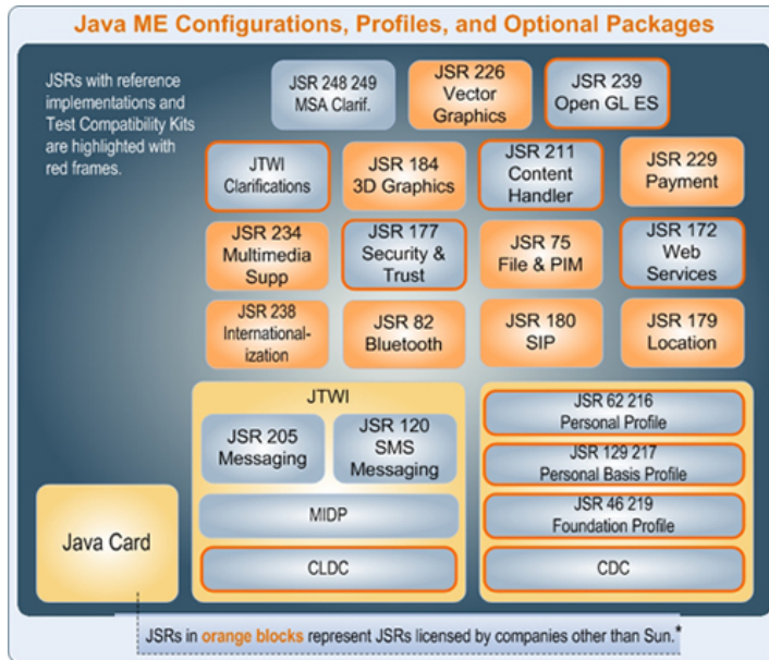
Obr. 6-3: Konfigurace, profily a volitelné balíčky Java ME (Zdroj: http://developers.sun.com/mobility/getstart/ )
