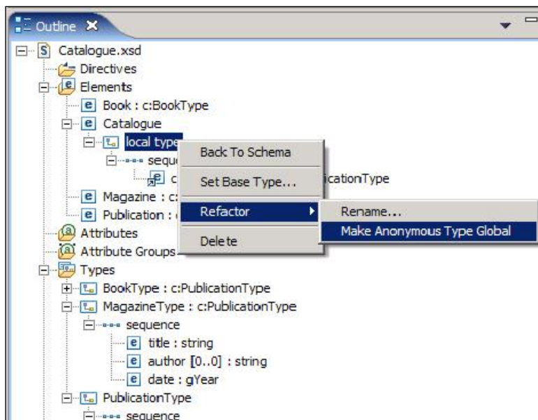
Obr. 1-10: Jednoduchost refaktoringu s podporou Eclipse IDE (použití refaktorovací metody Rename... )
