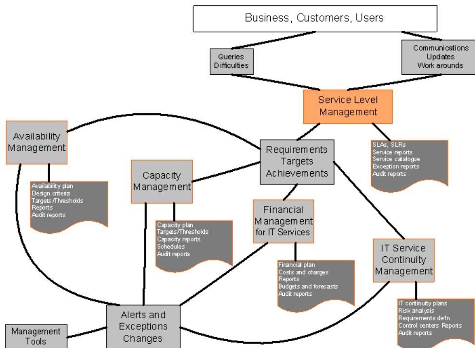
Obr. 4-7: ITIL® procesy pro Service Delivery (zdroj: ITIL).
