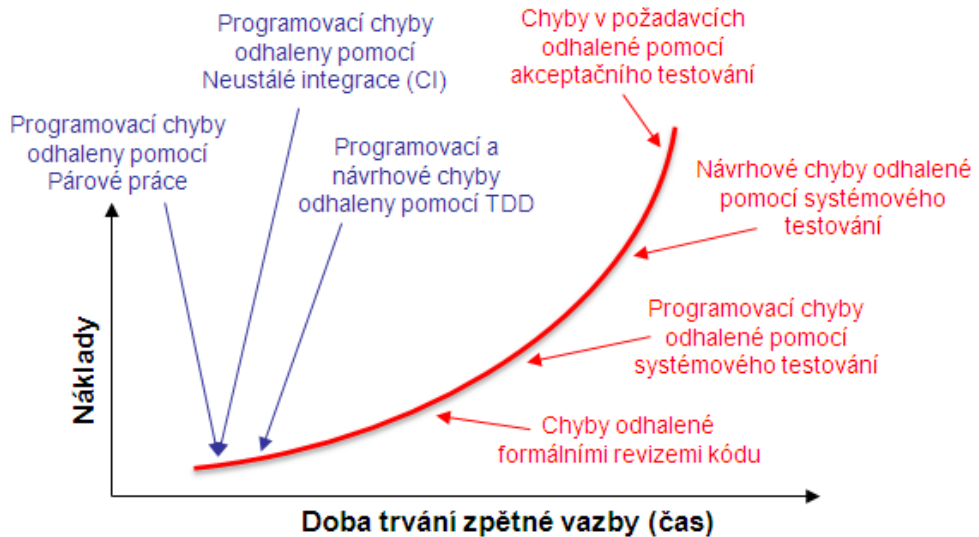
Obr. 1-9: Cena chyby v průběhu životního cyklu aplikace (červená křivka) a techniky minimalizující cenu opravy chyby v různých fázích životního cyklu aplikace. Všimněte si ceny TDD (zdroj [Am06]).
