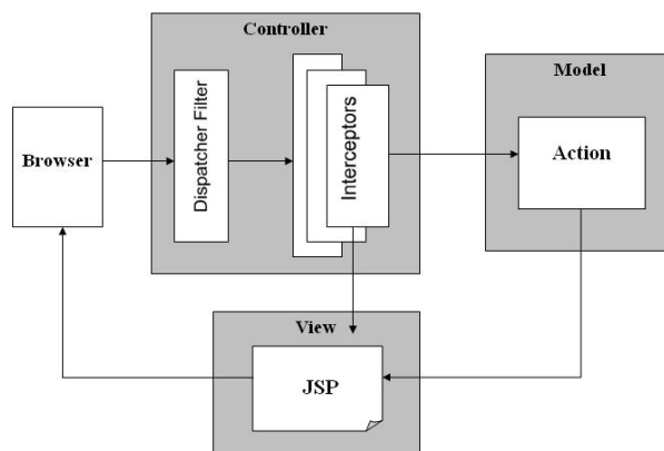
Obr. 6-26: Architektura Struts 2 (Zdroj: http://www.javaorigin.com )
