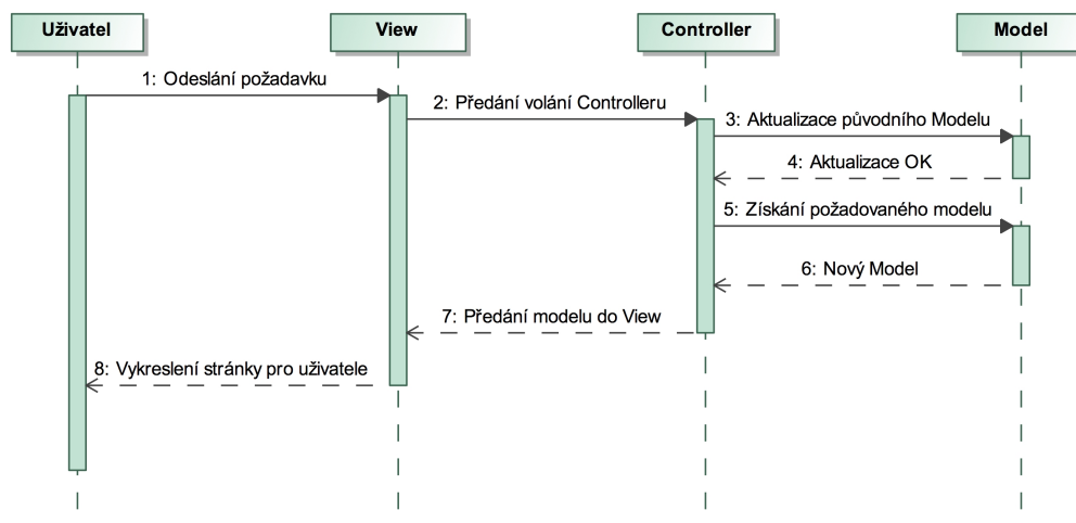
Obr. 9-5: Sekvenční diagram návrhového vzoru MVC
