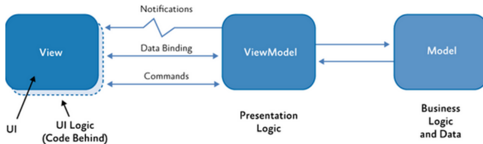
Obr. 9-9: Schéma návrhového vzoru Model View View Model
