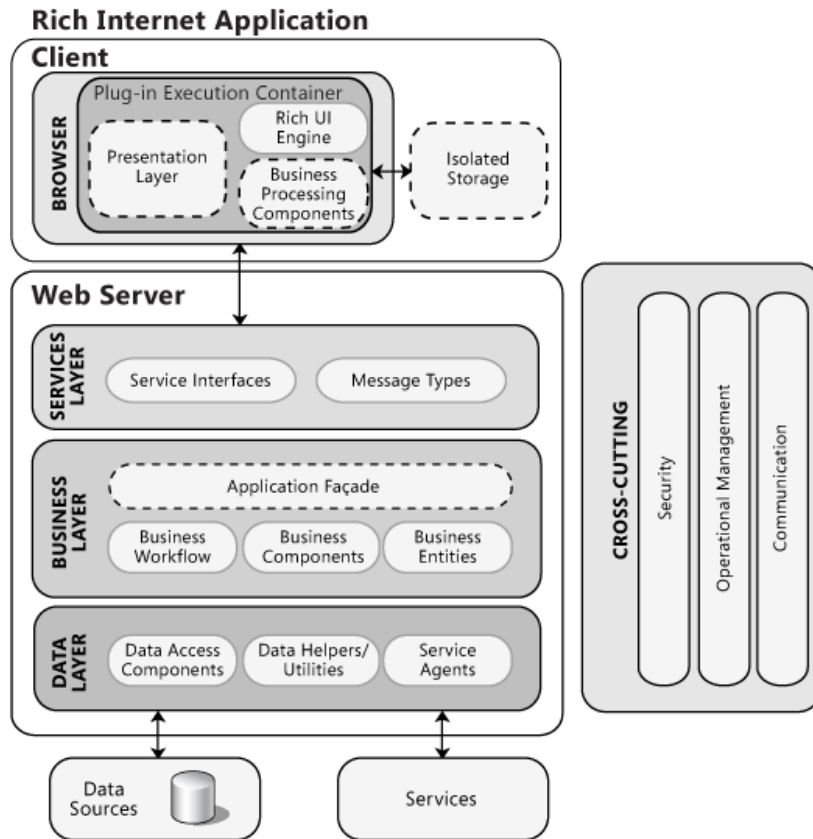
Obr. 9-2: Architektura webové aplikace - Rich Internet Application
