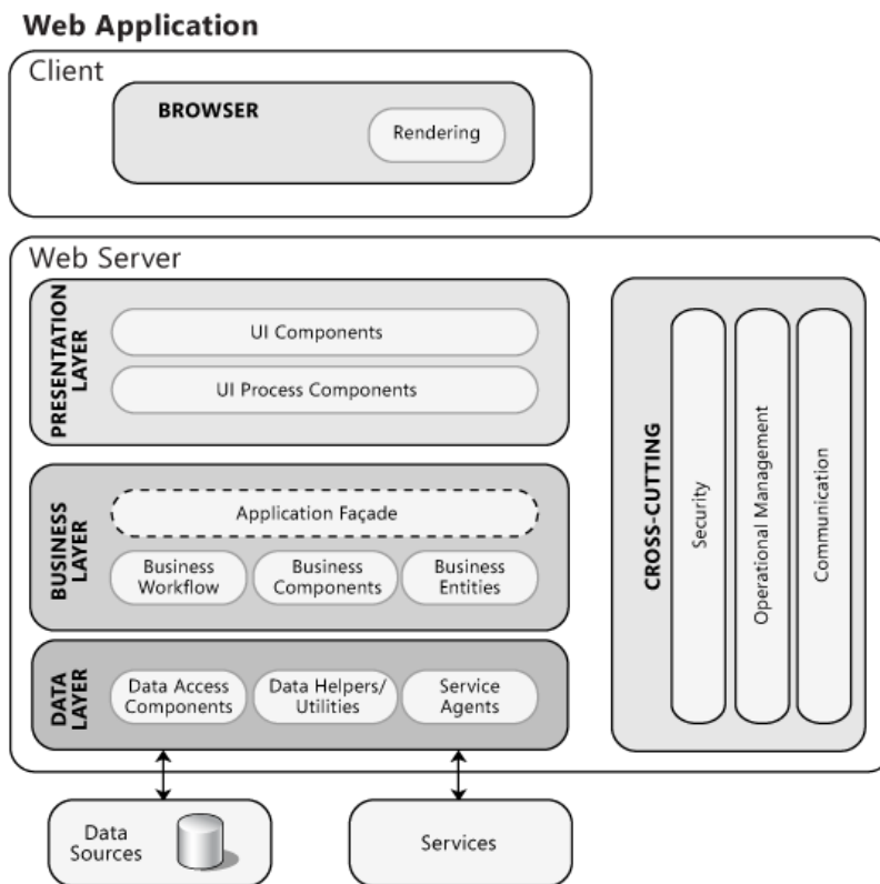
Obr. 9-1: Architektura webové aplikace - klasický přístup
