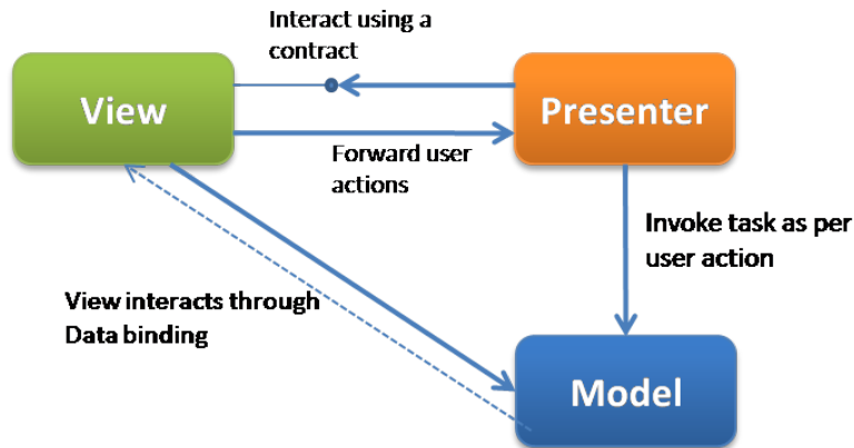
Obr. 9-7: Schéma návrhového vzoru MVP - Supervising Controller
