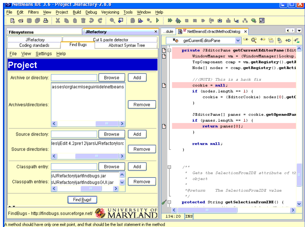
Obr. 1-11: Nástroj JRefractory 4 a hlášení o chybě – metoda má mít pouze jedno místo návratu včetně zvýraznění oněch několika míst (zdroj: vlastní).
