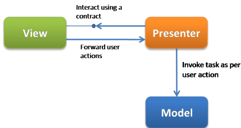
Obr. 9-6: Schéma návrhového vzoru MVP - Passive View
