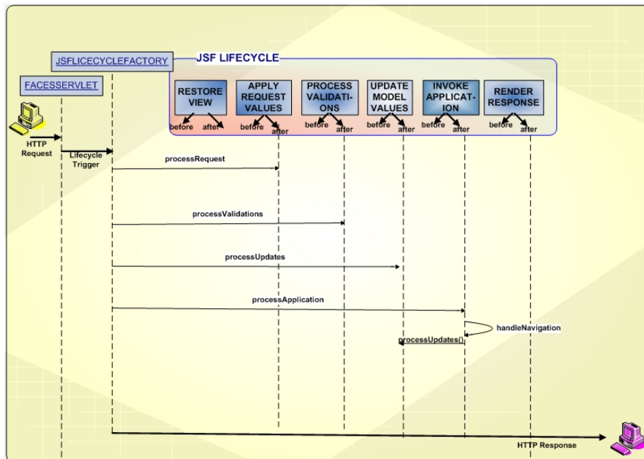
Obr. 6-27: Životní cyklus JSF (Zdroj: http://www.javaworld.com )
