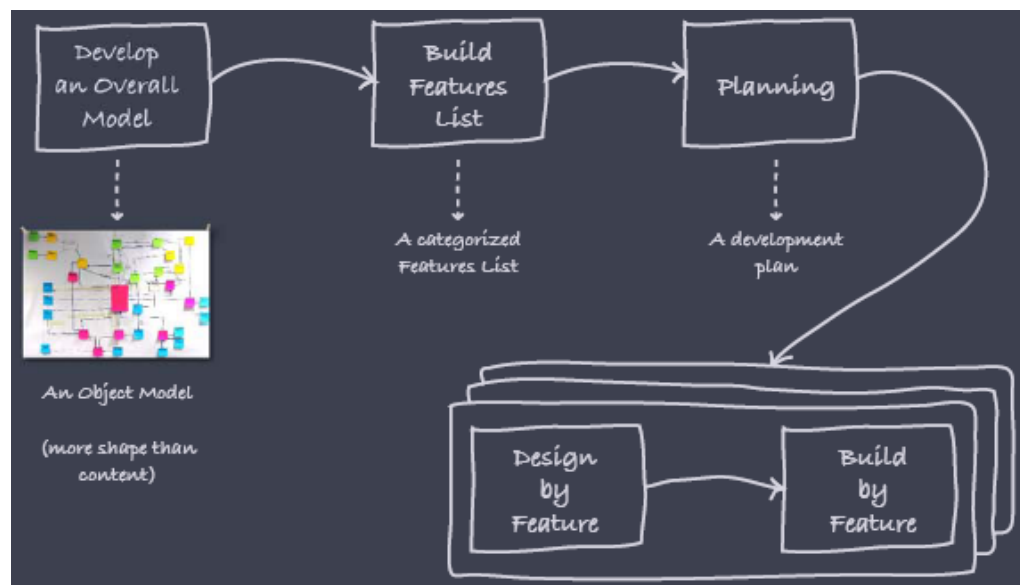
Obr. 1-7: Aktivity FDD a jejich sled (zdroj: [Lu05])
