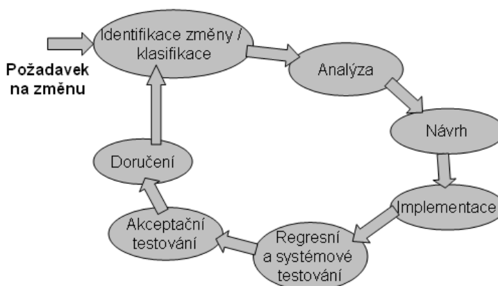
Obr. 4-9: Proces údržby podle IEEE 1219.
