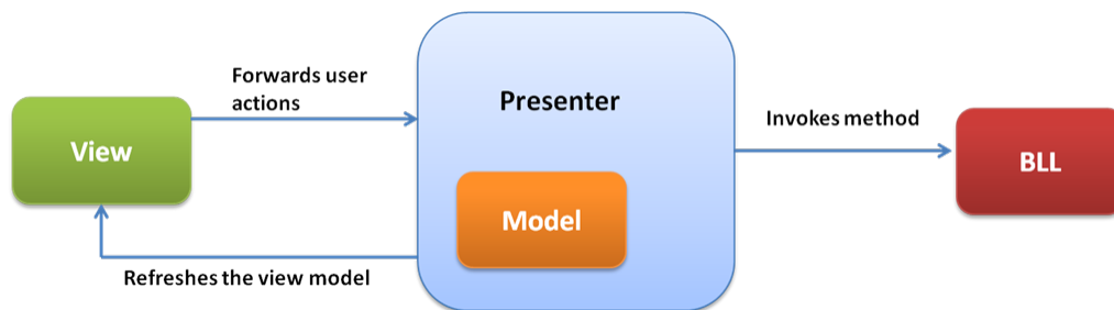
Obr. 9-8: Schéma návrhového vzoru Presenter-Model
