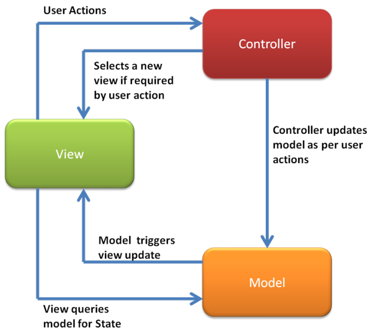
Obr. 9-4: Schéma návrhového vzoru MVC
