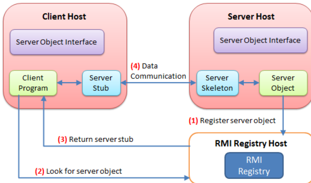
Obr. 6-9: RMI ve čtyřech krocích (Zdroj: http://lycog.com/distributed-systems/ )
