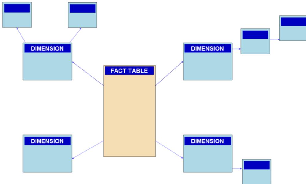
Obr. 12-4: Snow flake schéma
