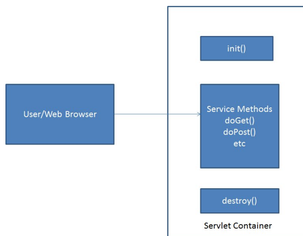
Obr. 6-12: Životní cyklus servletu (Zdroj: http://inheritingjava.blogspot.cz )
