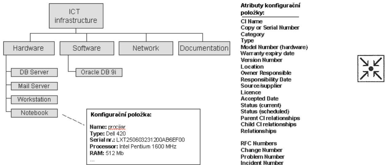
Obr. 4-6: Struktura konfiguračních položek, příklad atributů.
