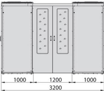
Vorderansicht
