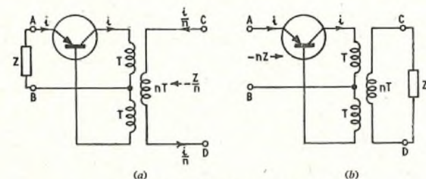
FIG. 4—NEGATIVE-IMPEDANCE CONVERTOR
