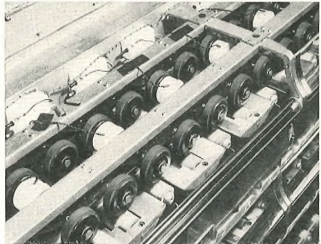
FIG. 9—IDLING ROLLERS
