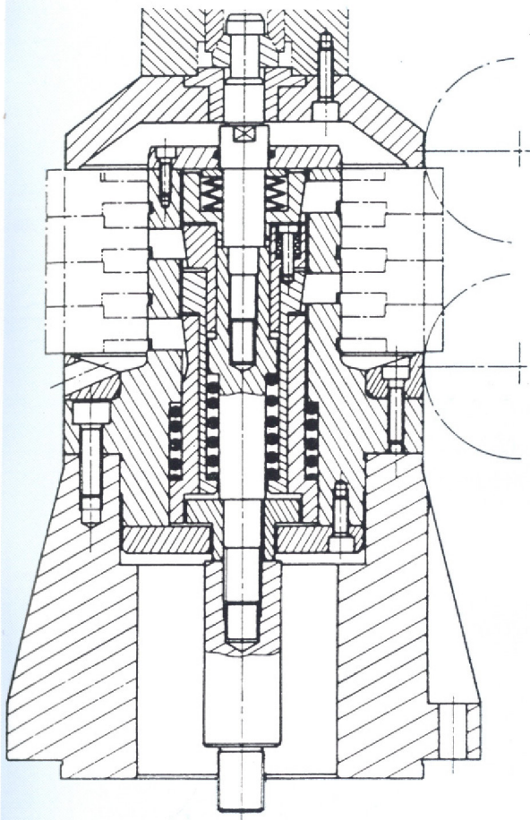
ESEMPI DI MANDRINI CON "TASSELLI AD ESPANSIONE"
