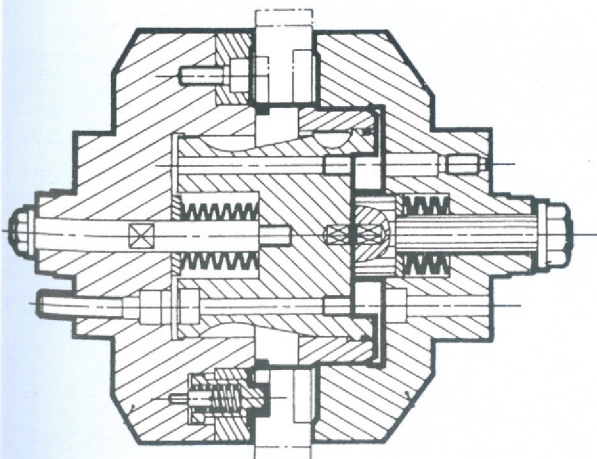
Mandrini per lavorazioni di sbaratura
