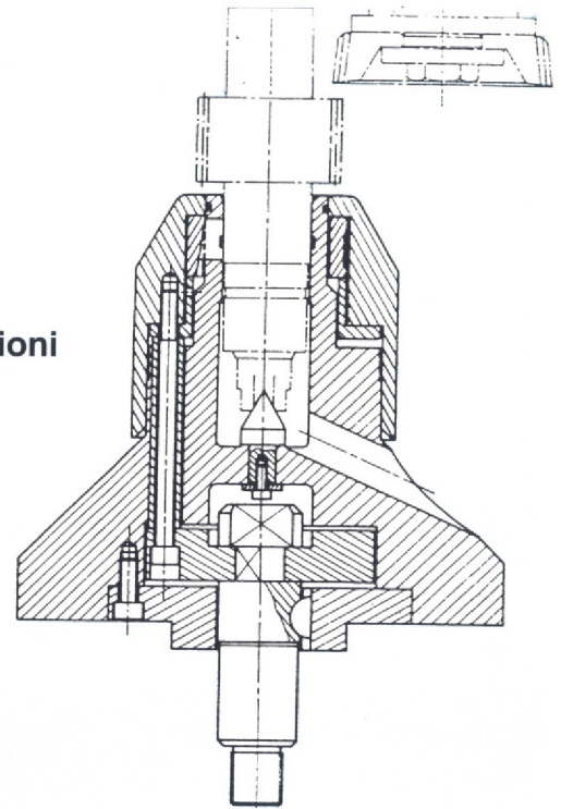
ESEMPI DI MANDRINI CON "TASSELLI AD ESPANSIONE"
