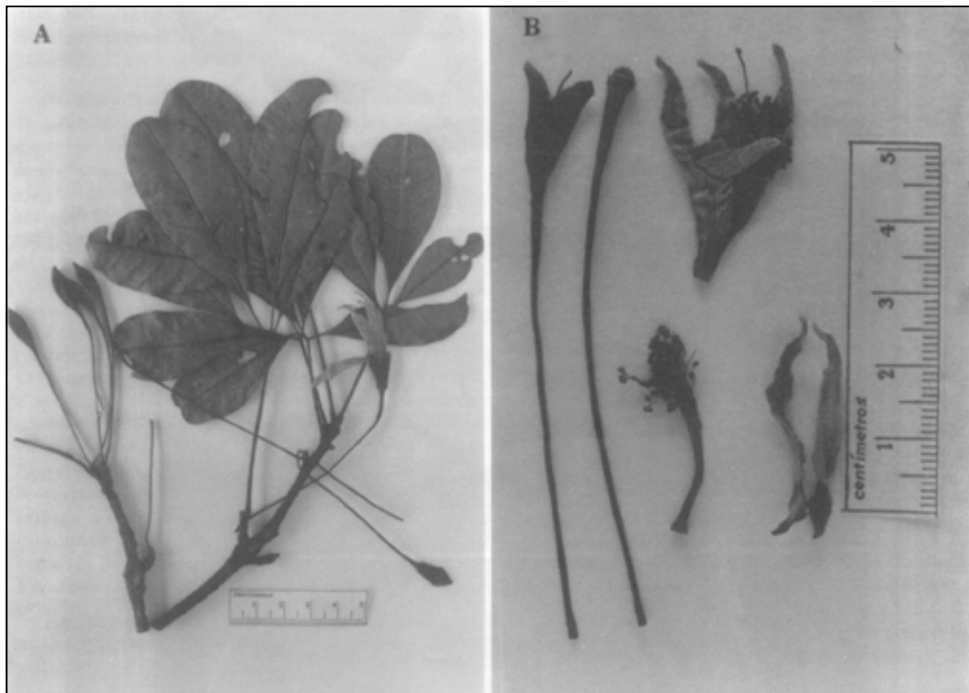
Figura 3. Eriotheca lorentensis Fern. Alonso. A. Rama con botones florales y una flor abierta. B- Detalles de la flor (pedicelo, cáliz, corola y columna estaminal). (Fotografiado de la serie típica C. Grández, I. Hudson & N. Jaramillo 4964).
