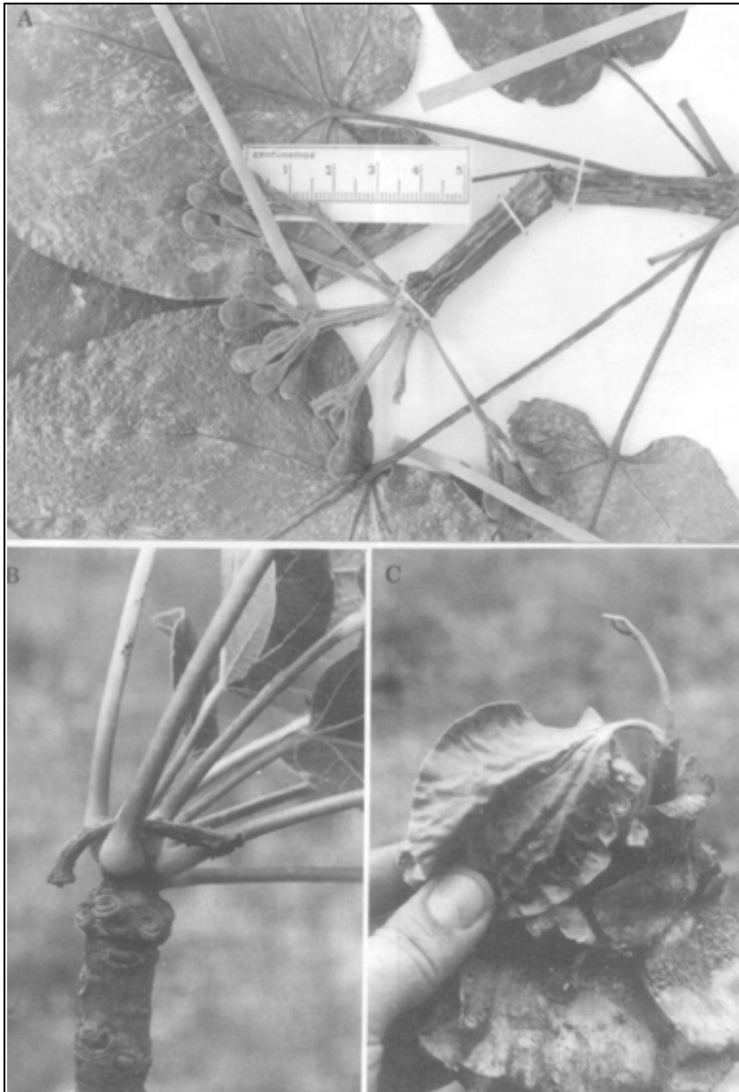
Figura 2. Cavanillesia chicamochaе Fern. Alonso. A. Rama con inflorescencia terminal (con botones florales), fotografiado de Albesiano 725 (COL); B- Detalle de un ápice de rama, mostrando las cicatrices foliares (Fotografiado de la serie típica Fernández-Alonso 19938, COL). C- Detalle de una plántula con los restos de la sámara (Fotografiado de la serie típica).
