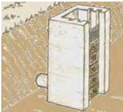
Photo J. Premier étage du moine associé à la première buse (Guinée) [© APDRA-F] (CIRAD).
