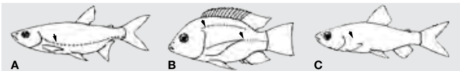
Figure 165. Ligne latérale. A : Complète ; B : Interrompue sur deux niveaux ; C : Incomplète.
