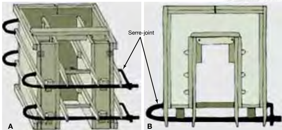
Figure 88. Moine de moine. A : Vue de face ; B : Vue de dessus.
