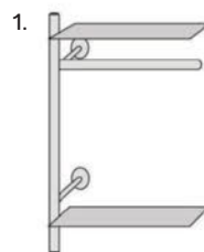
Garderobenelement (B 80 cm) 1 x Kleiderstange 2 x Boden
