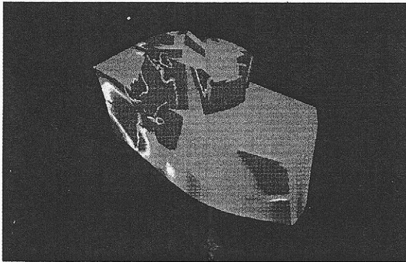
3.60. Guggenheim Museum : Gaussian analysis.
