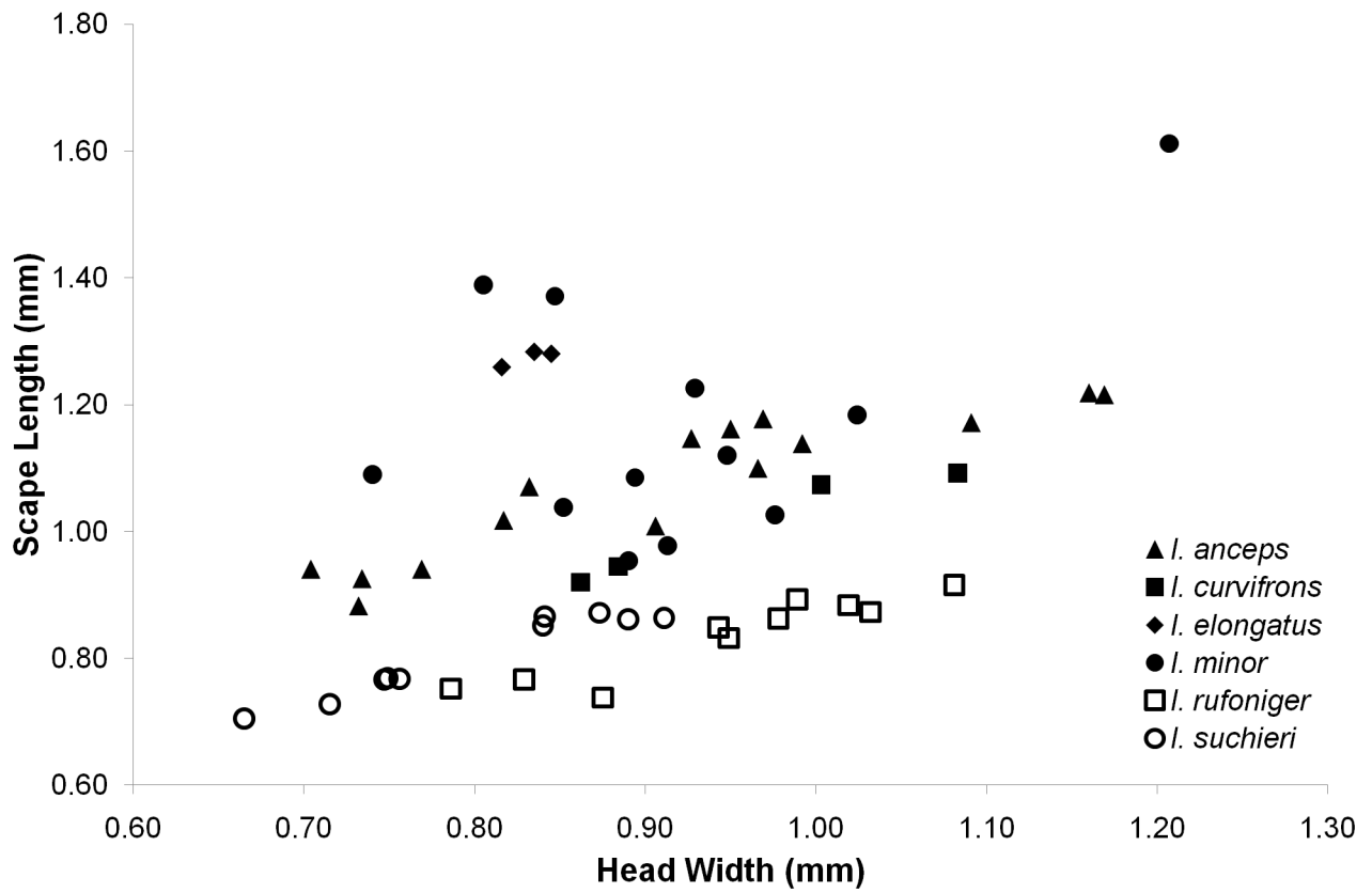
FIGURE 92. Scape length versus head width for I. anceps , I. curvifrons , I. elongatus , I. minor , I. rufoniger and I. suchieri .
