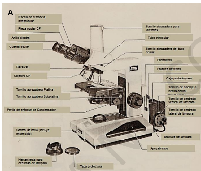
Descripción (ejemplo) de microscopio óptico. A) Vista lateral derecha. B) Vista lateral izquierda.
