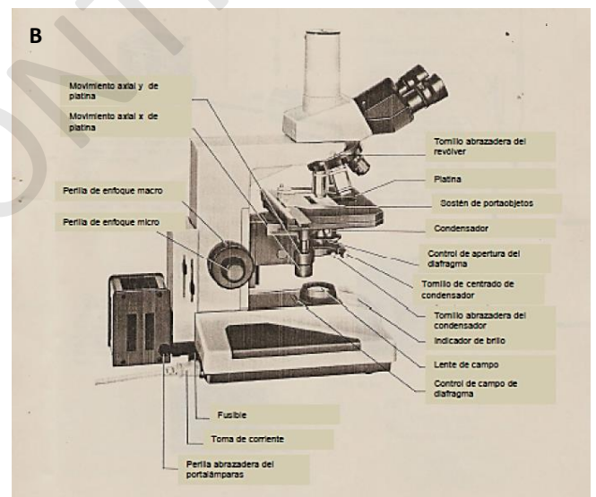
Descripción (ejemplo) de microscopio óptico. A) Vista lateral derecha. B) Vista lateral izquierda.
