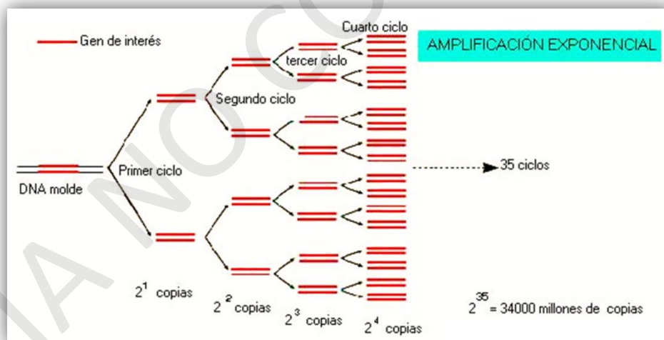
Amplificación exponencial de la PCR
