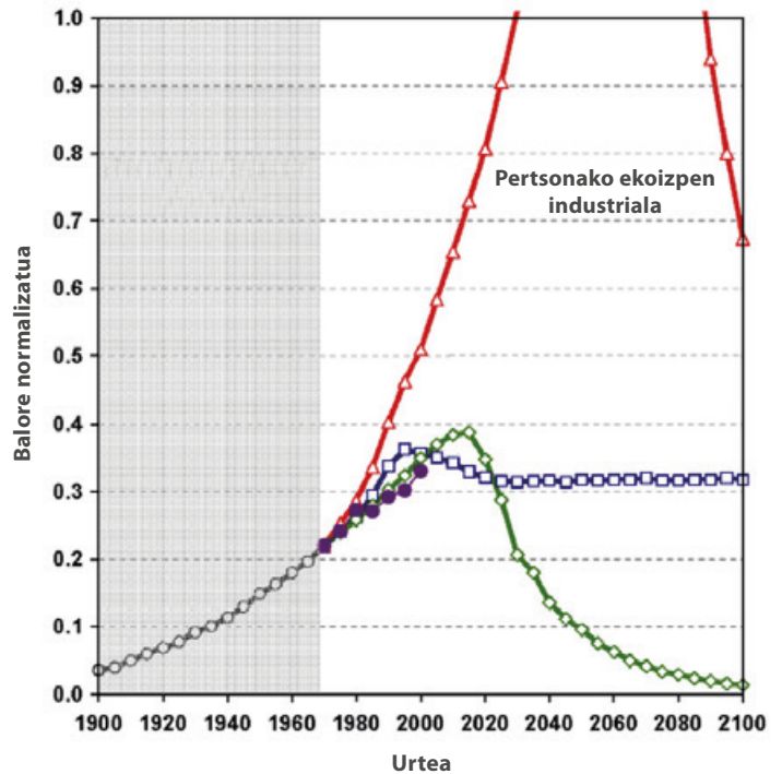
—■— Mundu egonkortua —▲— Hobekuntza teknikak —◇— Oinarrizko hipotesia —○— "Limits to Growth" txosteneko emaitza —●— Behaketak
