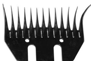
Wellington Untermesser Feinwollkamm besonders geeignet für Merinos 13 Zähne, Bevel 7 mm, Scherbreite 93 mm
