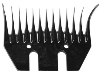
Wellington Untermesser für die schnelle Schur geeignet für geübte Scherer 13 Zähne, Bevel 5 mm, Scherbreite 94 mm
