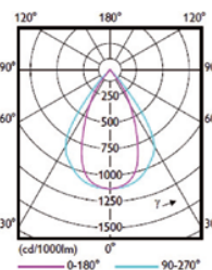
Engstrahlend (NB)
