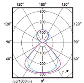
SP402P, direkt-indirekt
