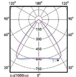
SM530C, BAP-tauglich
