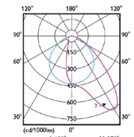
SP544P, asymmetrisch
