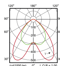
DA25W (Doppelt asymmetrisch breitstrahlend, 25°)
