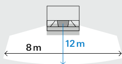
Busch-Wächter® 110 MasterLINE.
