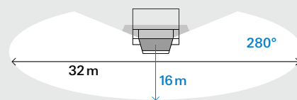
Busch-Wächter® 280 MasterLINE.
