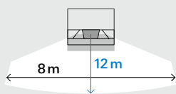
Busch-Wächter® 70 MasterLINE.
