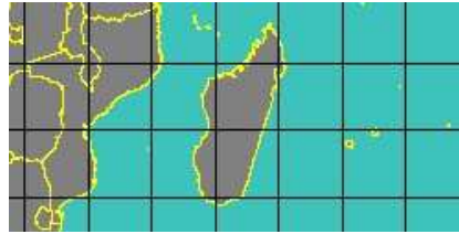
5220000515 Tropidophora boucheti E. Fischer-Piette, P. Blanc, F. Blanc, & F. Salvat, 1993 Madagascar
